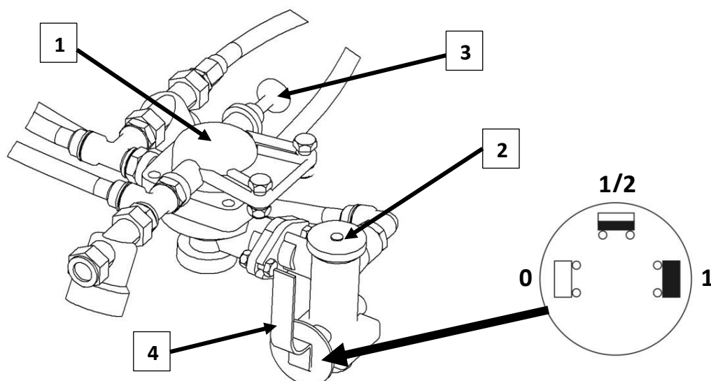
Rys. 4.14. Pneumatyczny regulator siły hamowania.
