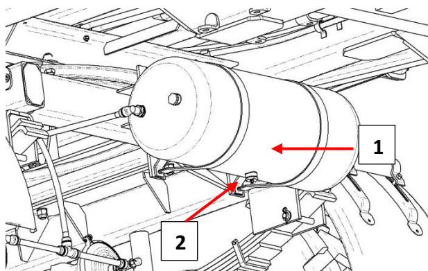
Rys. 6.5 Odwadnianie zbiornika powietrza
