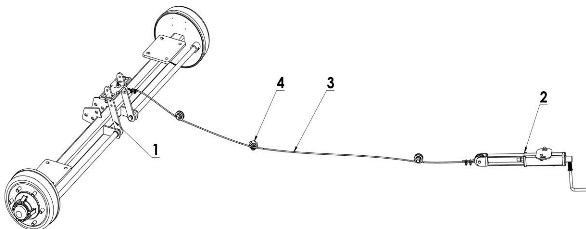
Rys. 4.15 Hamulec postojowy z mechanizmem korbowym
