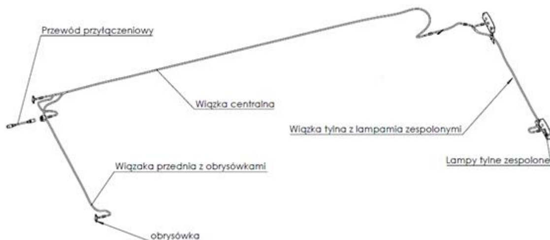
Rys. 4.16. Schemat instalacji elektrycznej rozrzutnika -standard
