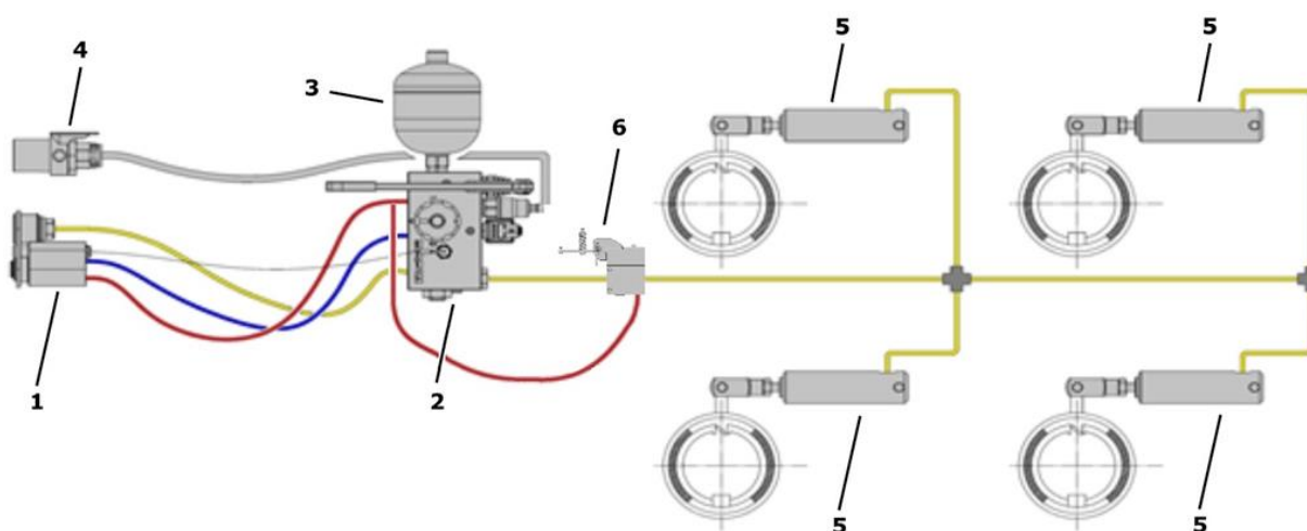
Rysunek 4.13. Schemat hydraulicznej instalacji hamulcowej.
