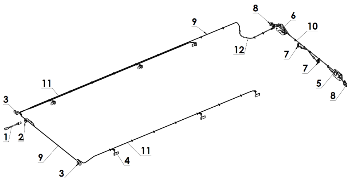
Rysunek 4.17 Schemat instalacji elektrycznej rozrzutnika z podświetlanymi lampami obrysowymi bocznymi (opcja)
