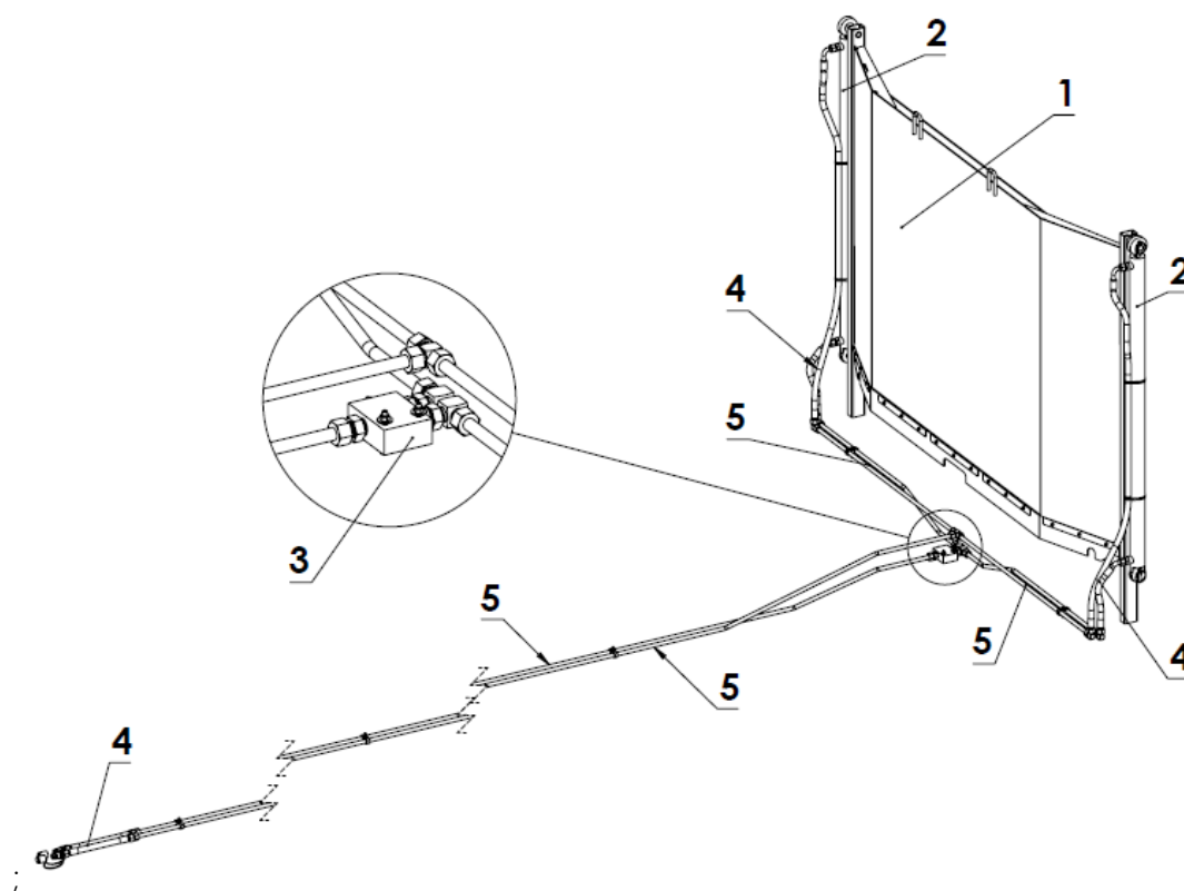
Rysunek 4.8. Budowa ściany tylnej hydraulicznej
