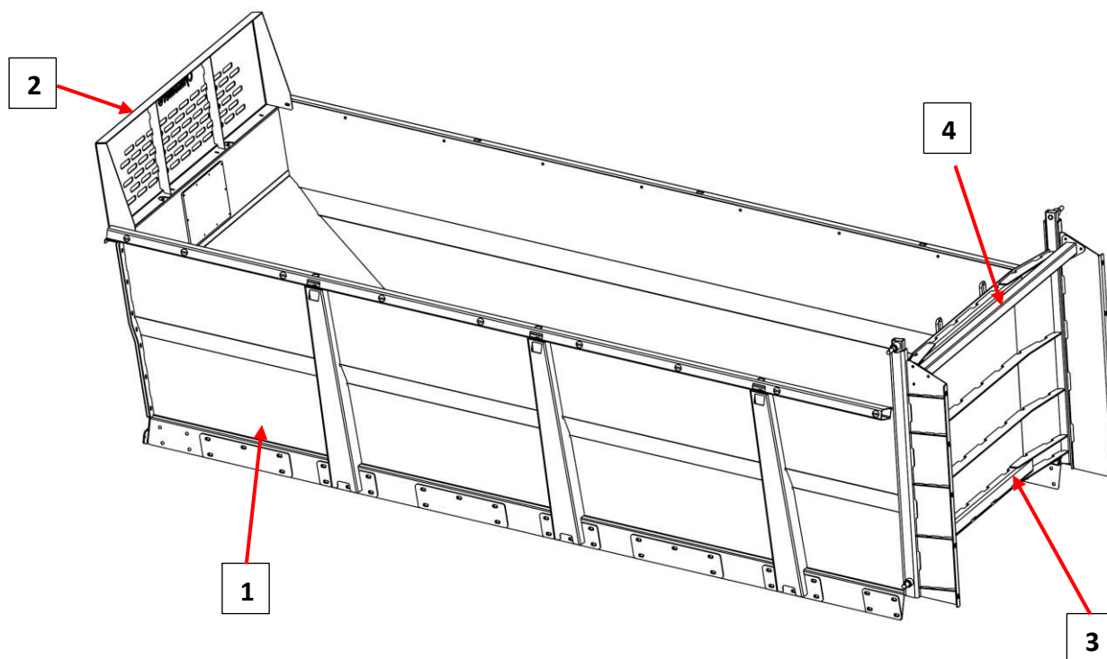
Rysunek 4.5. Skrzynia rozrzutnika
