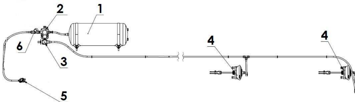
Rysunek 4.10. Schemat pneumatycznej instalacji hamulcowej jednoprzewodowej z ręcznym regulatorem siły hamowania.
