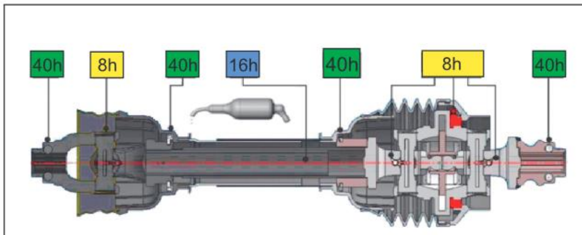
Rysunek 6.8. Częstotliwość smarowania wału przegubowego
