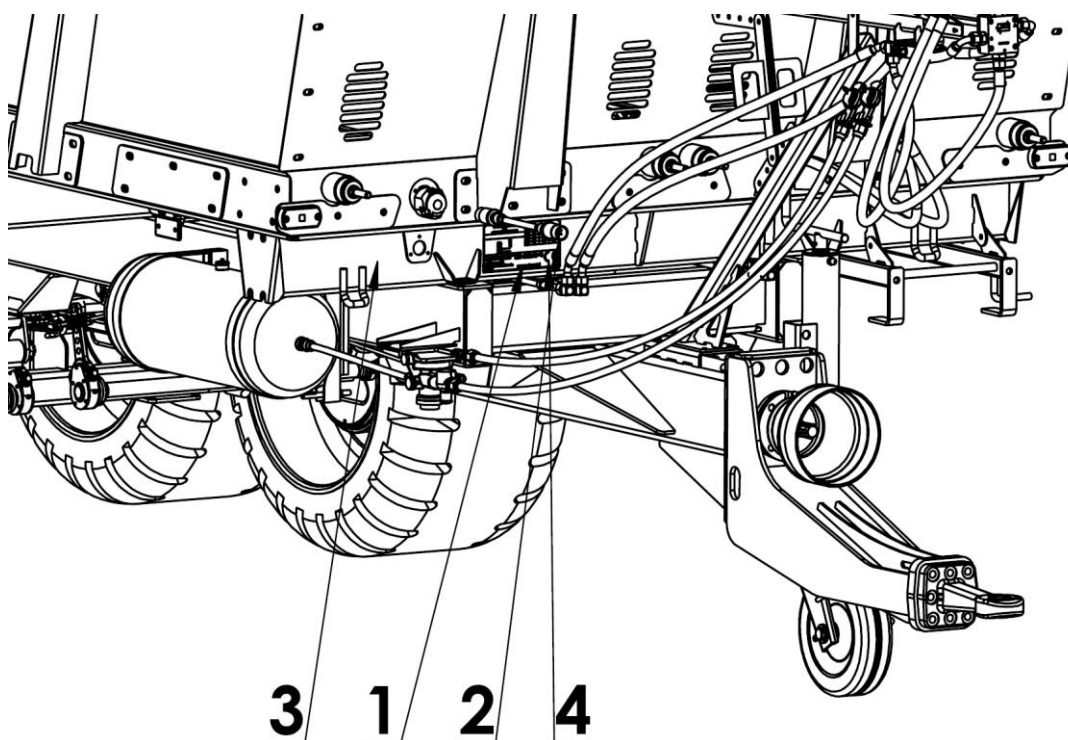
Rysunek 1. Możliwe miejsce umieszczenia tabliczki znamionowej i wybicia numeru fabrycznego, oraz wzór tabliczki znamionowej
