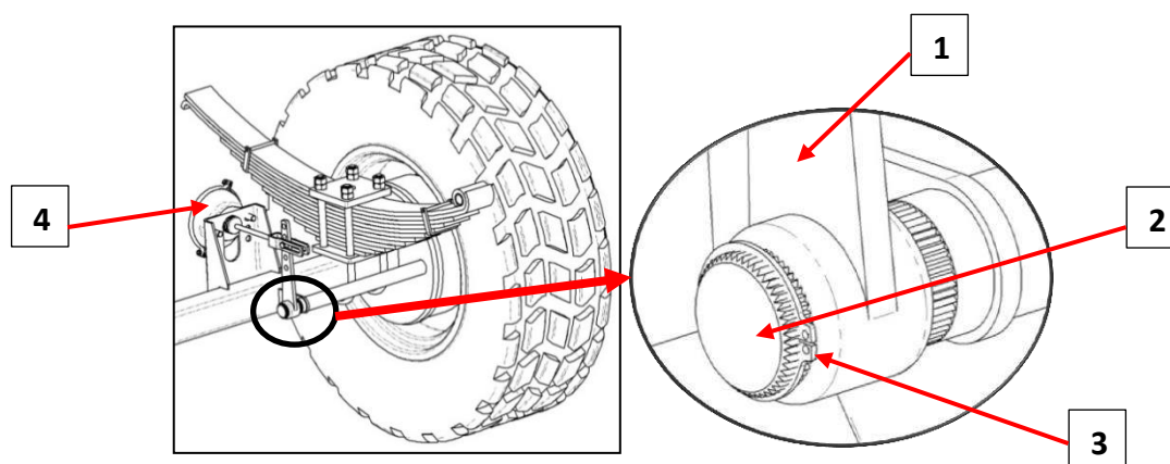
Rysunek 6.3. Regulacja hamulców
