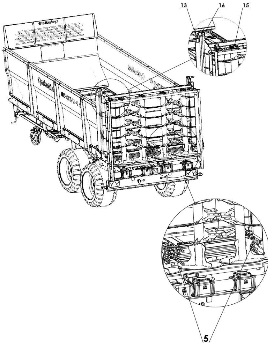
Rys. 6.7. Punkty smarowania rozrzutnika N-221/3-4
