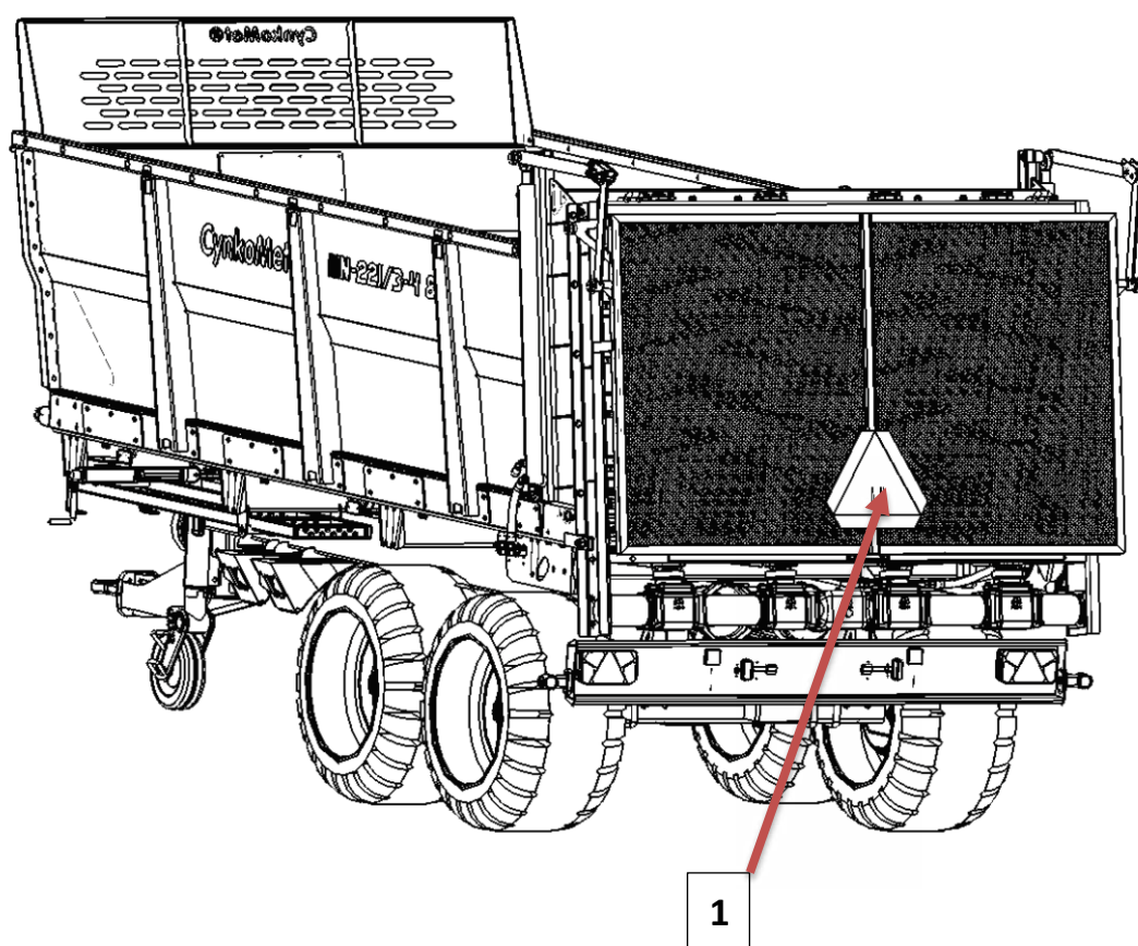
Rysunek 3.2. Miejsce umieszczenia tablicy wyróżniającej pojazdy wolno poruszające się.
