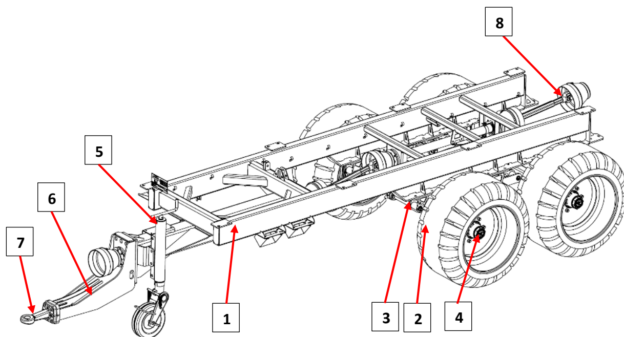
Rys. 4.2 Podwozie rozrzutnika
