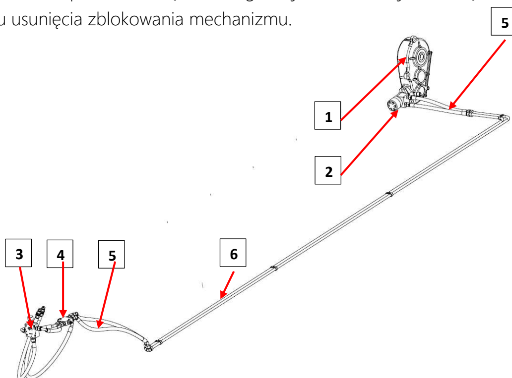
Rysunek 4.7. Budowa napędu przenośnika
