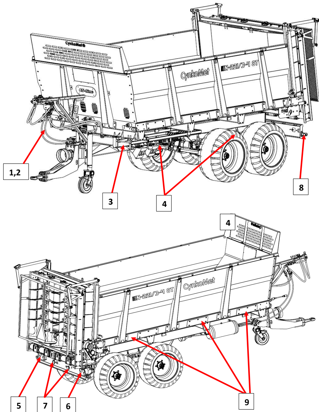
Rysunek 4.18. Schemat układu oświetlenia i sygnalizacji
