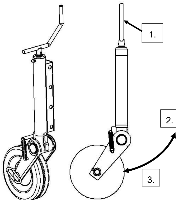
Rysunek 4.19 Regulowana podpora (od lewej: izometria, rzut z boku).
