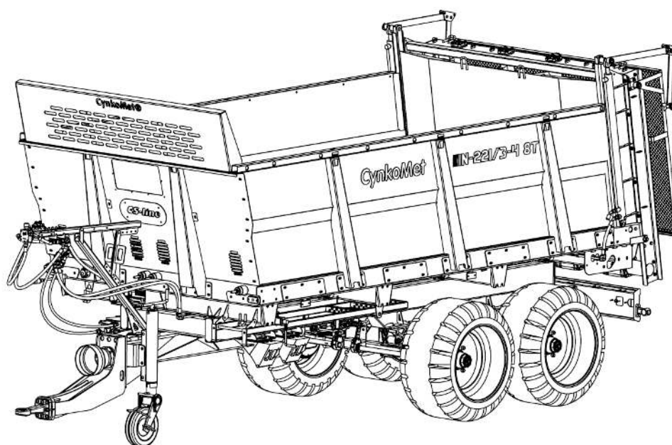
Rys. 4.1 Rozrzutnik N-221/3-4 CS-line
