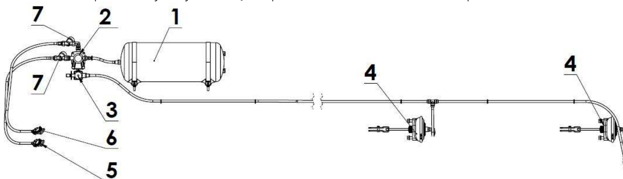
Rysunek 4.11. Schemat pneumatycznej instalacji hamulcowej dwuprzewodowej z ręcznym regulatorem siły hamowania.
