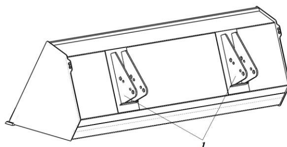
Рисунок 3 – Ковш 0,8 м 3 (для КУН(TURS)-1000Y): 1 – пластина с кронштейнами
