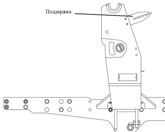
Рисунок 5 – Панель навески для КУН1000У-0БС
