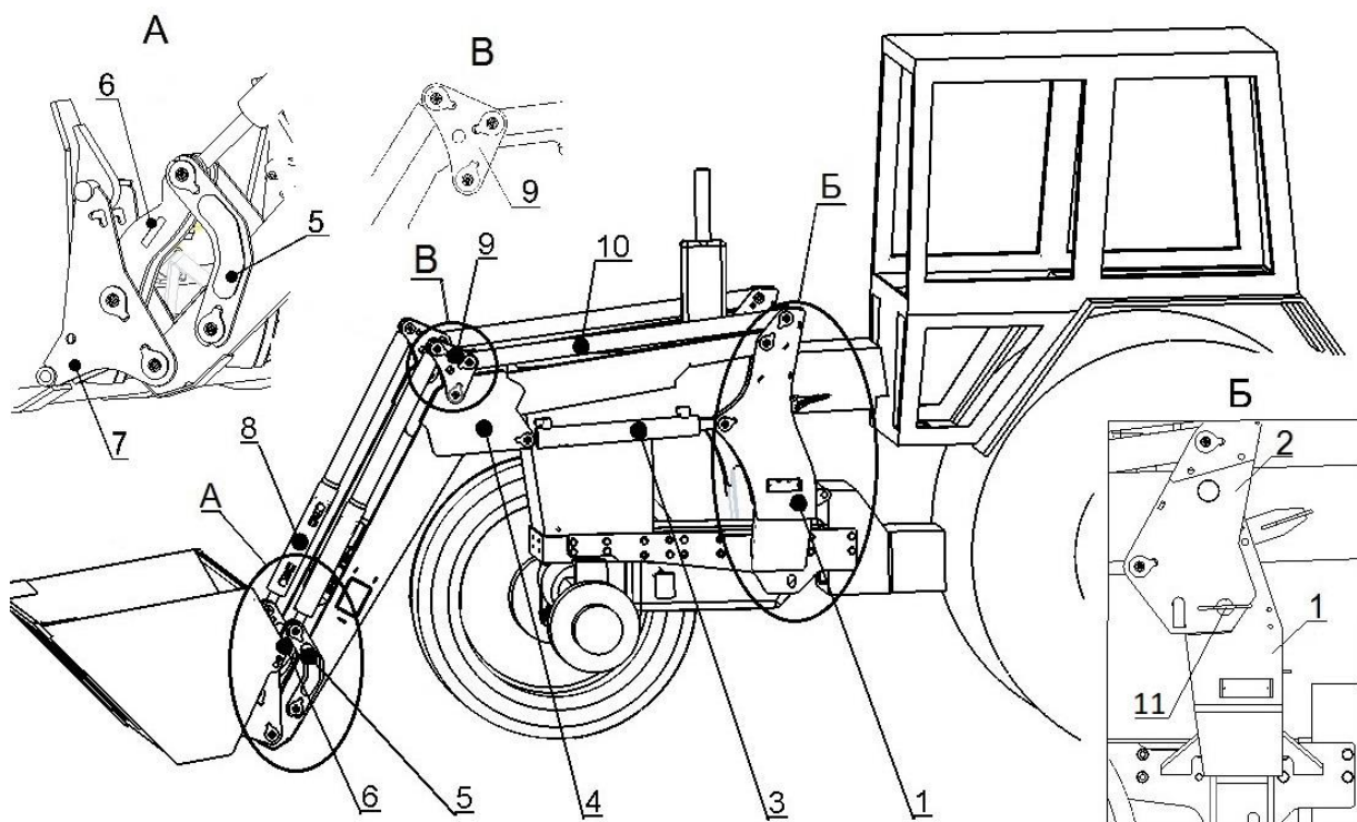
Рисунок 1 – Общий вид погрузчика КУН(TURS)-1000Y-0 с ковшом 0,8м 3 (вид А – для погрузчиков КУН(TURS)-1000Y-0П и КУН(TURS)-1000Y-0БС; вид Б – для погрузчика КУН(TURS)-1000Y-0БС):
