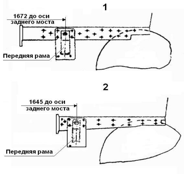
Рис.15. Места крепления передней рамы
