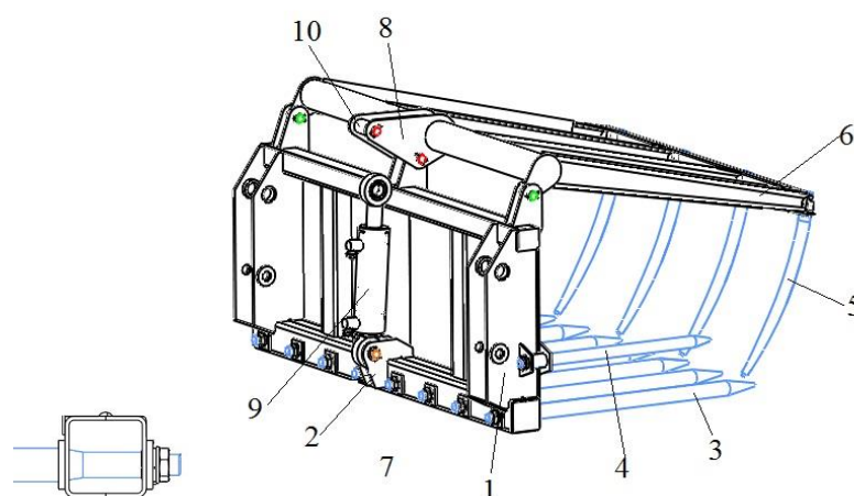
Рис. 12. Вилы
