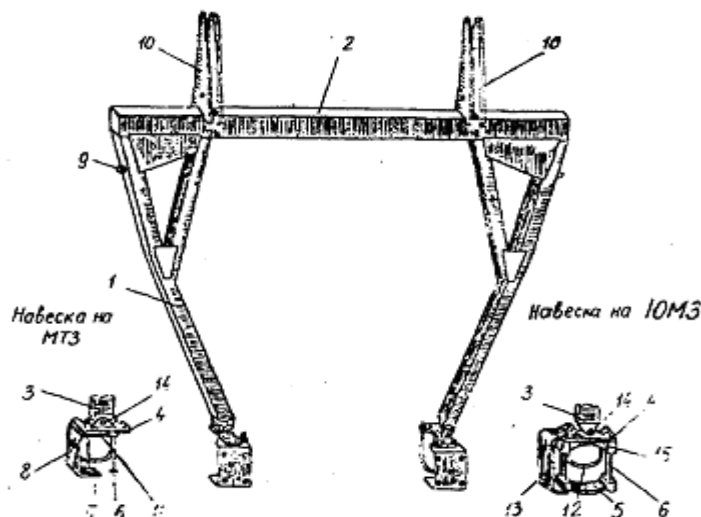
Рис. 4. Рама опорная
