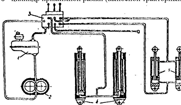
Рис. 23. Принципиальная схема гидросистемы при работе с ковшом:
