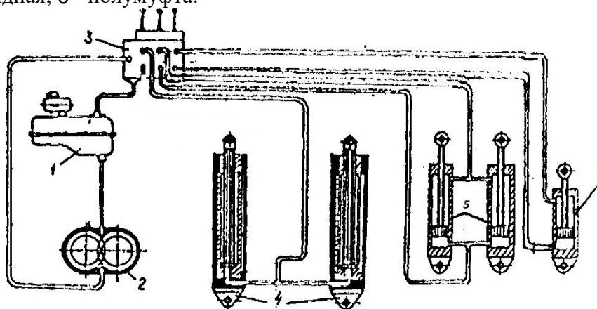
Рис. 22. Принципиальная схема гидросистемы при работе с вилами:
