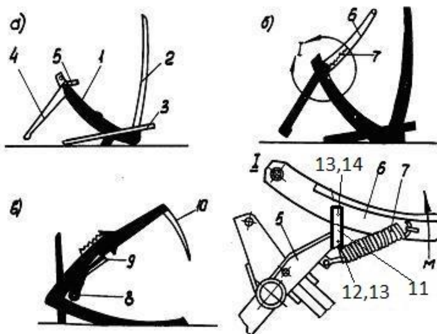
Рис. 19. Порядок сборки гребельной решетки:
