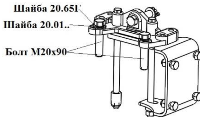
Рис. 4А
