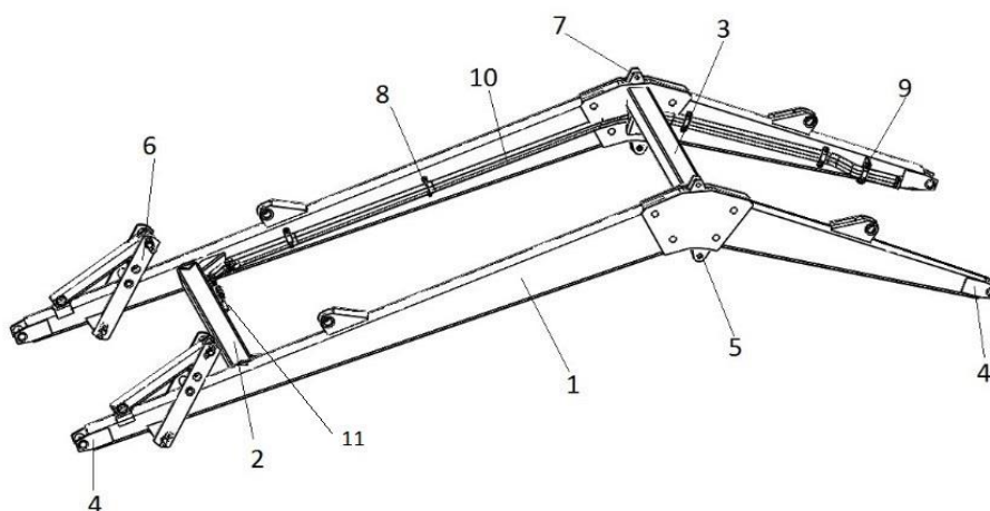
Рис. 5. Рама подъема
