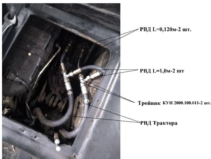
Рис. 24. Присоединение РВД кабине тракторов типа МТЗ:
