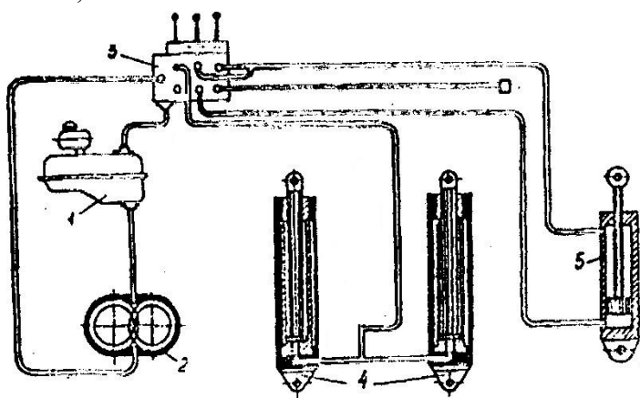
Рис. 20. Принципиальная схема гидросистемы при работе с платформой, установленной на раме подъема:
