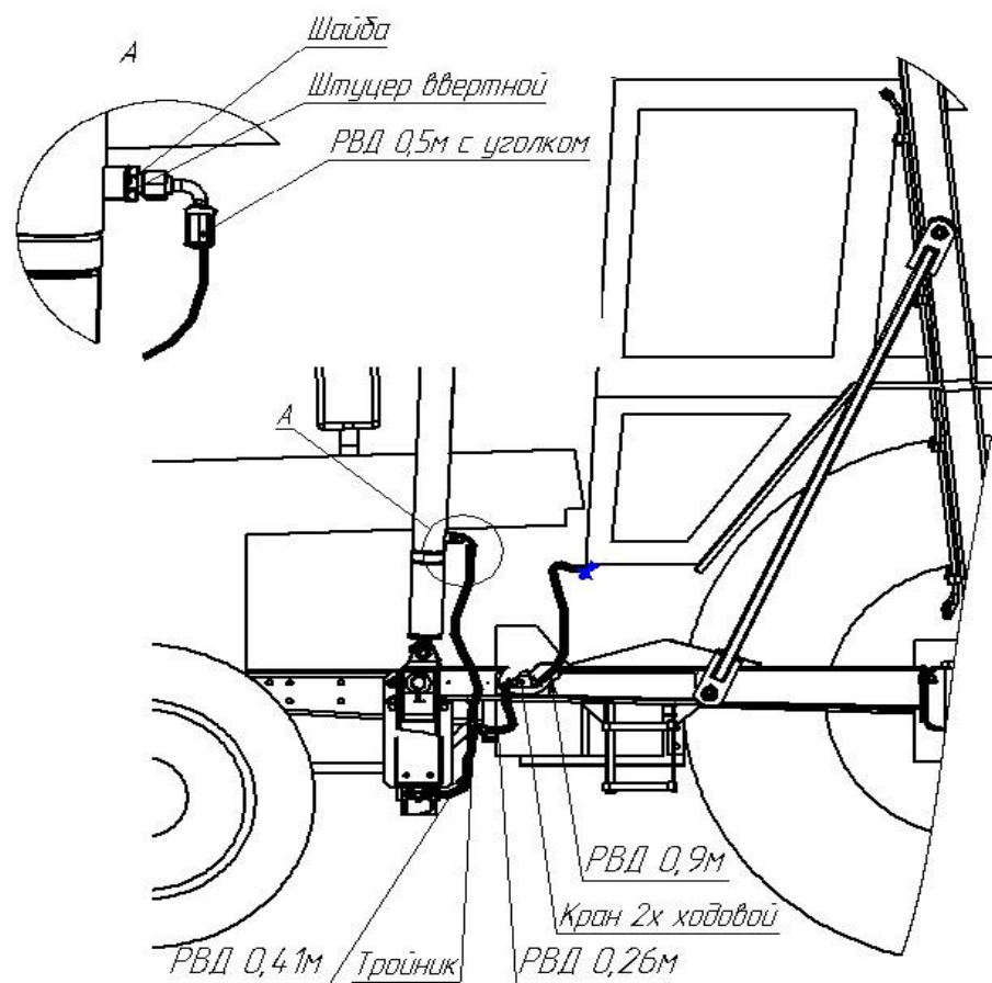
Рис. 16. Монтаж гидросистемы гидроцилиндров подъема.
