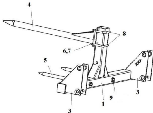
Рис. 13 а. Приспособление для погрузки рулонов
