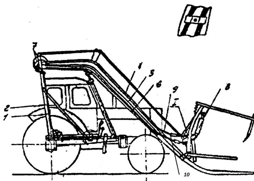
Рис. 17. Монтаж гидросистемы управления рабочими органами.
