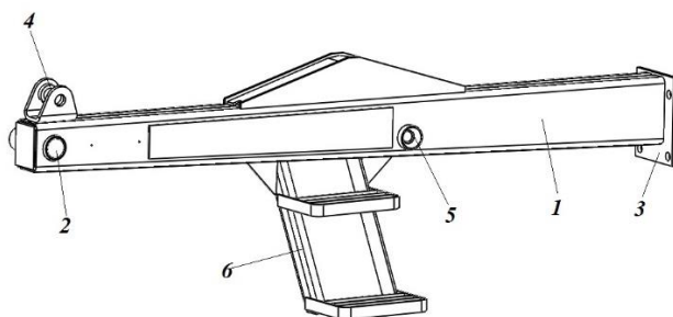
Рис. 6. Балка опорная левая
