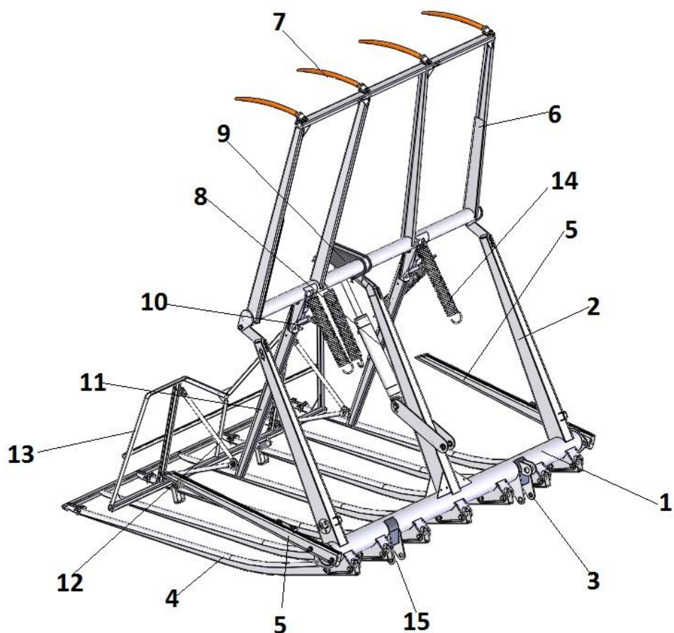
Рис. 10. Платформа.
