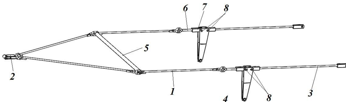
Рис. 8. Растяжка
