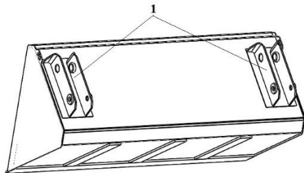
Рис. 13. Ковш 0,45м 3 для сыпучих грузов
