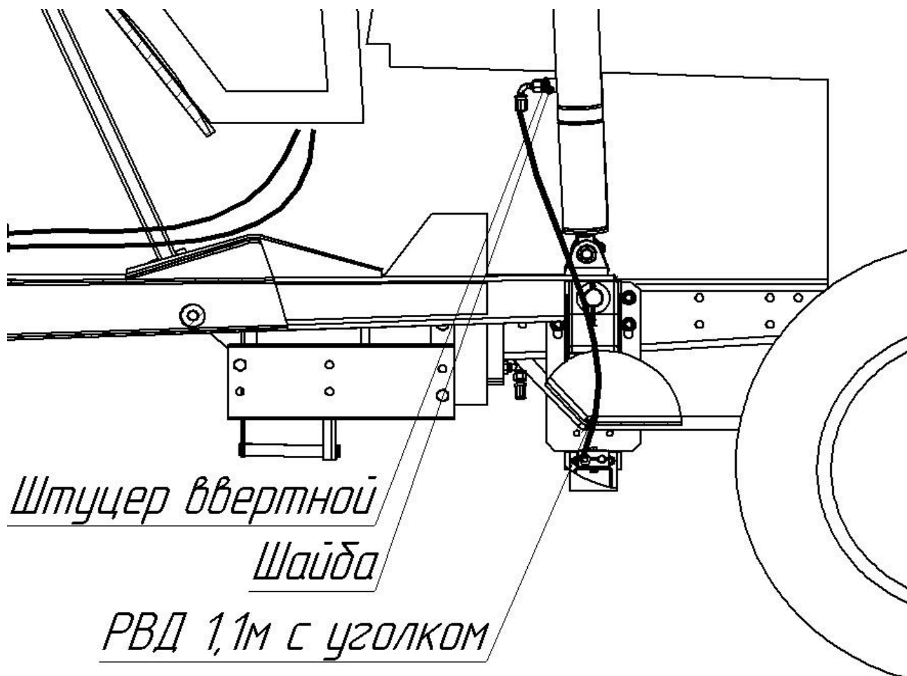
Рис.16А
