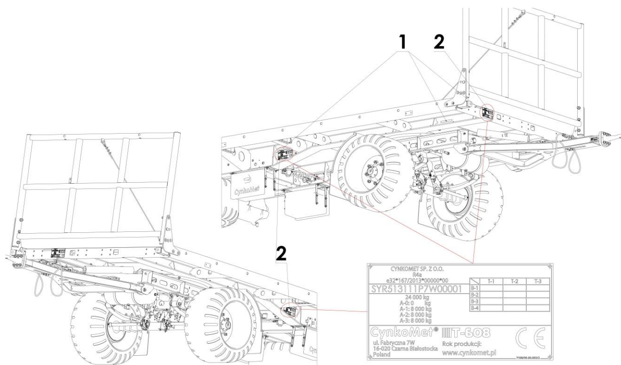
Rysunek 1. Miejsce umieszczenia tabliczki znamionowej i wybicia numeru fabrycznego 1 – możliwe miejsca wybicia numeru VIN, 2 – możliwe miejsca umieszczenia tabliczki znamionowej
