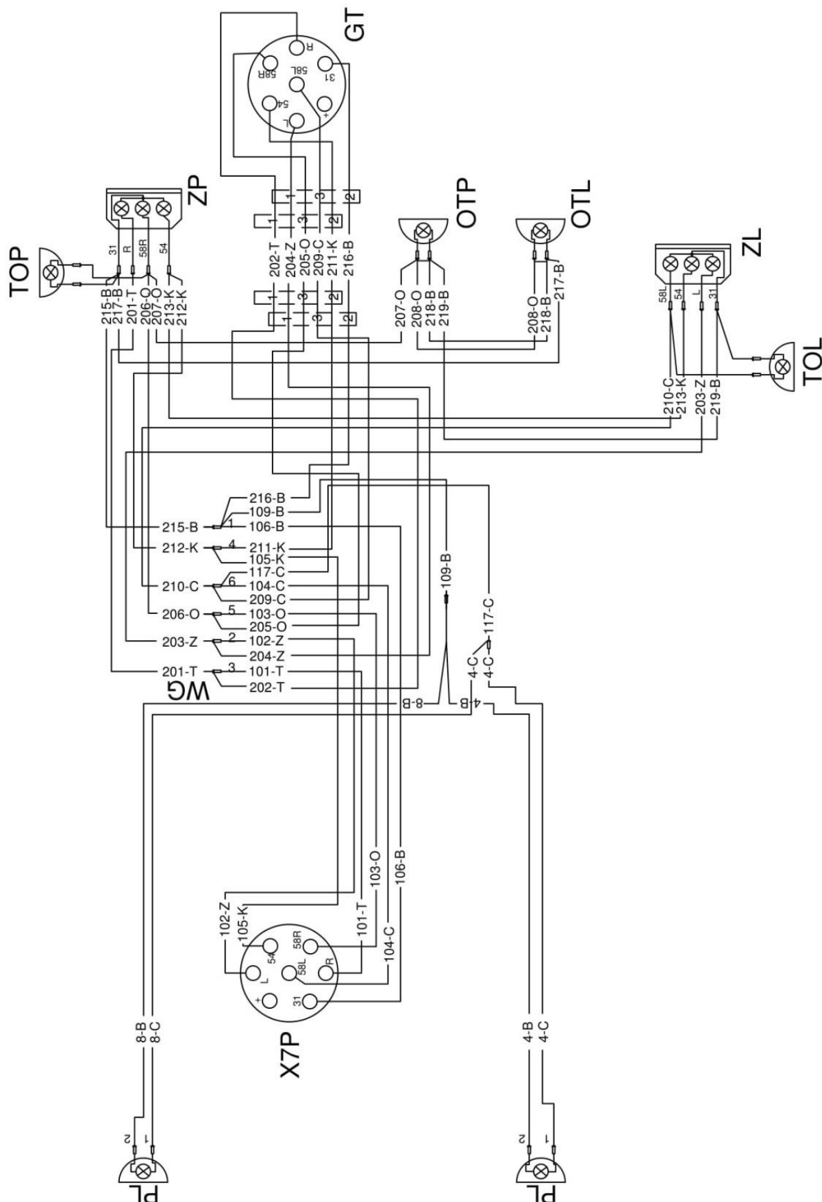
Rys. 9. Schemat instalacji elektrycznej przyczepy.
