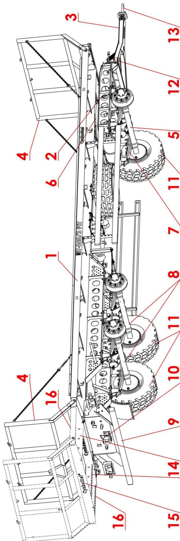
Rysunek 5. Podwozie przyczepy.
