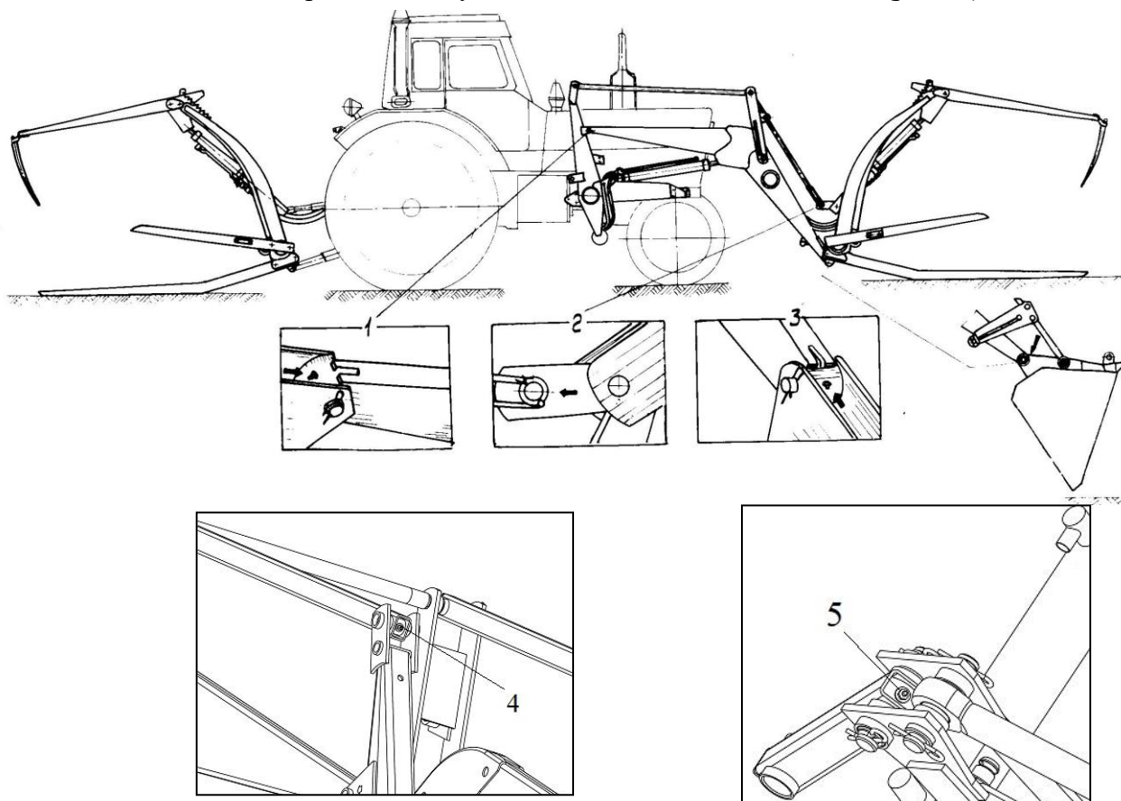
Рис.48 Схема смазки
