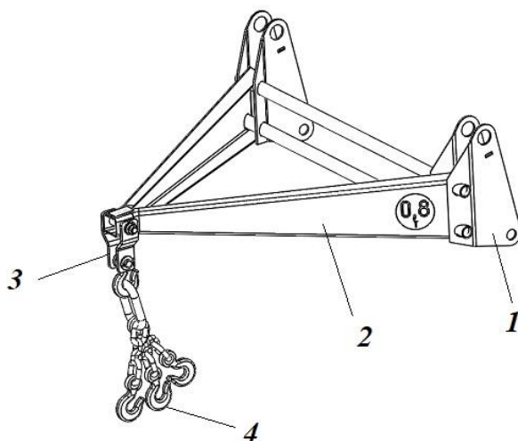
Рис. 14 Устройство грузоподъемное:
