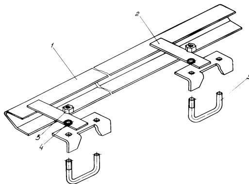
Рис. 11 Ограждение:
