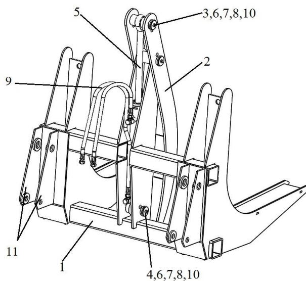
Рис.19 Бревнозахват
