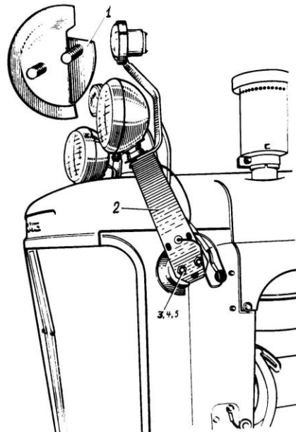
Рис. 25 Перестановка и крепление передних фар на тракторах ЮМЗ:
