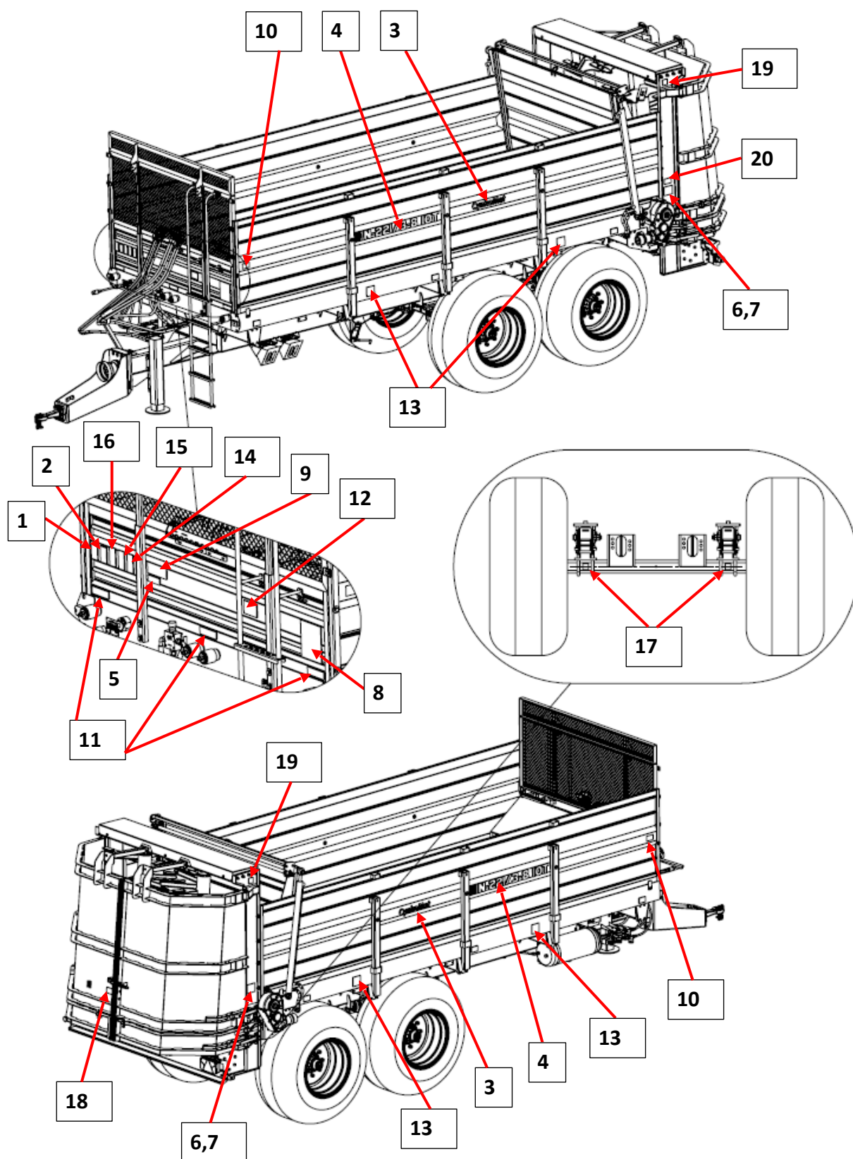
Rysunek 3.4. Rozmieszczenie naklejek.
