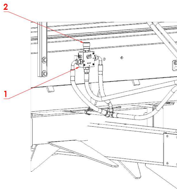
Rysunek 4.18. Regulacja prędkości przesuwu przenośnika podłogowego
