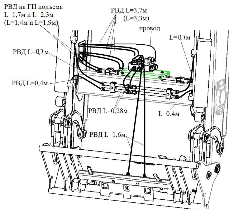
Рисунок 19 – Подсоединения РВД к дивертору для КУН(TURS)-1500-0Д и КУН(TURS)-2000-0Д
