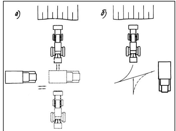
Рисунок 31 – Схема работы погрузчика: а – разгрузка при движении вперед и назад б – разгрузка при повороте погрузчика.
