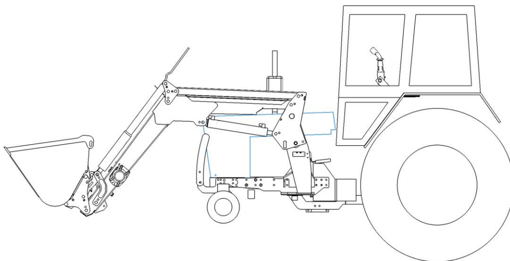
Рисунок 1В – Общий вид погрузчика КУН(TURS)-1200 с ковшом 0,8м 3
