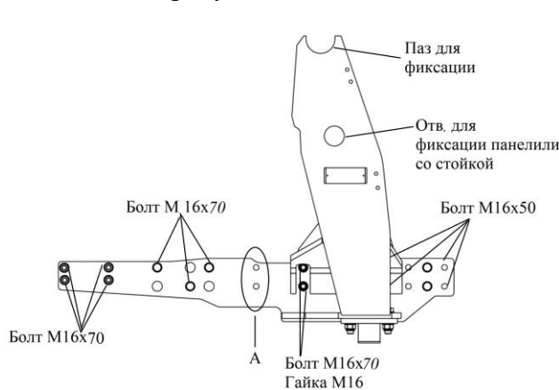
Рисунок 5 – Панель навески для КУН(TURS)-2000
