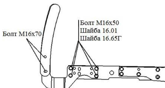
Рисунок 7Б – Ограждение для КУН(TURS)-1500
