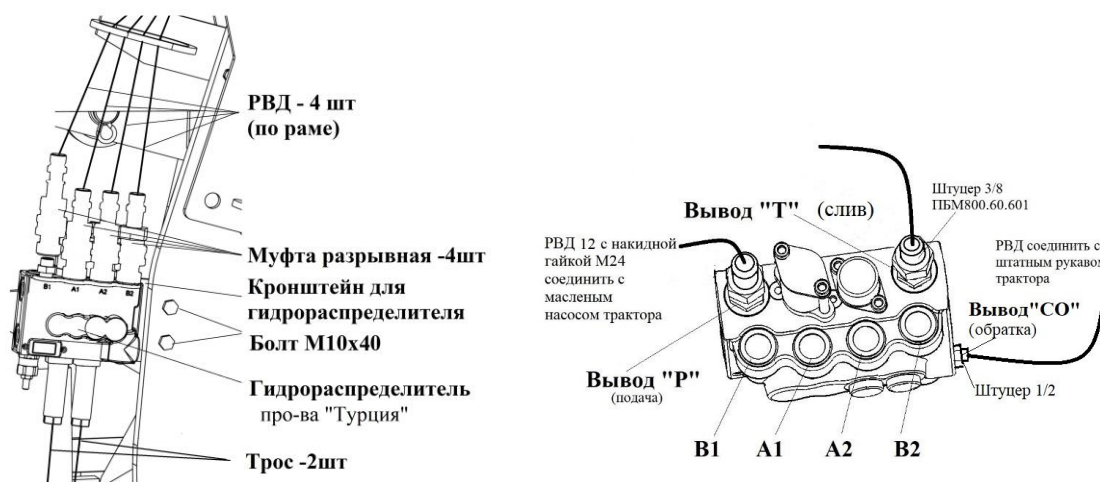
Рисунок 18 – Установка гидрораспределителя
