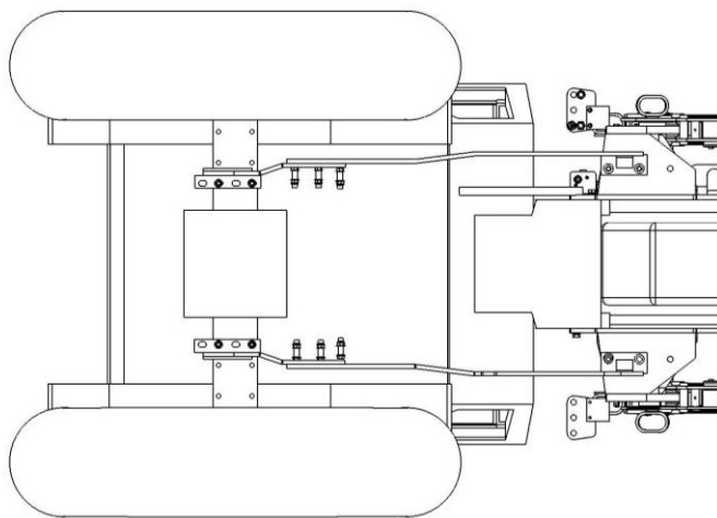
Рисунок 8Б – Установка разгружающих тяг на МТЗ-80/82 (вид снизу трактора)
