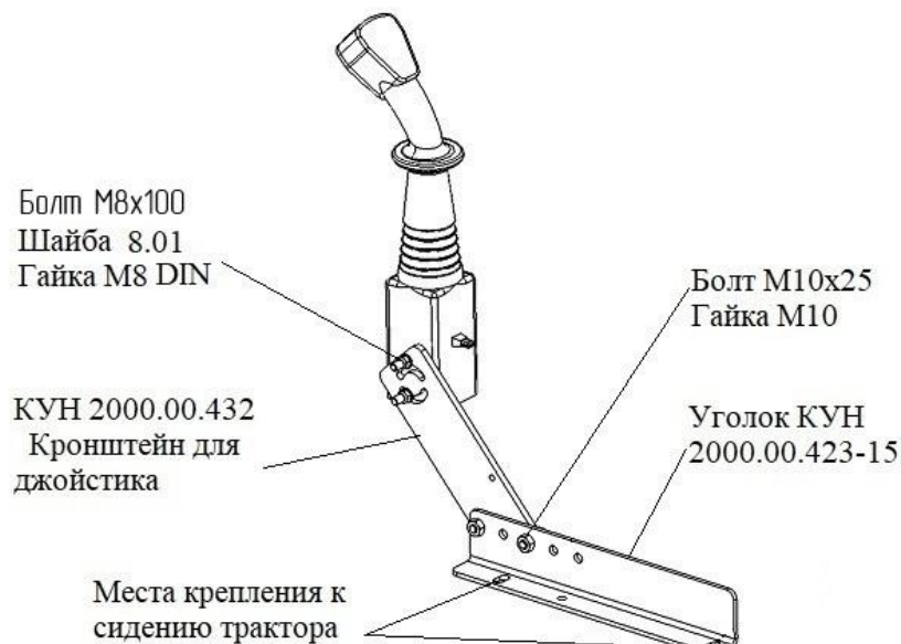
Рисунок 17 – Установка джойстика
