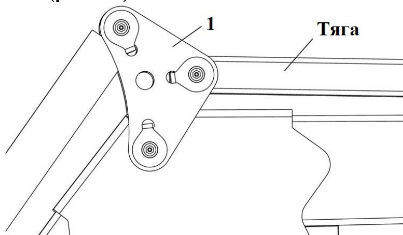
Рис.10А Установка кронштейна
