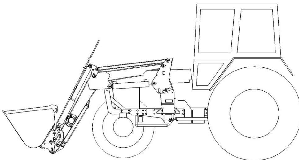
Рисунок 1Б – Общий вид погрузчика КУН(TURS)-1000 с ковшом 0,8м 3
