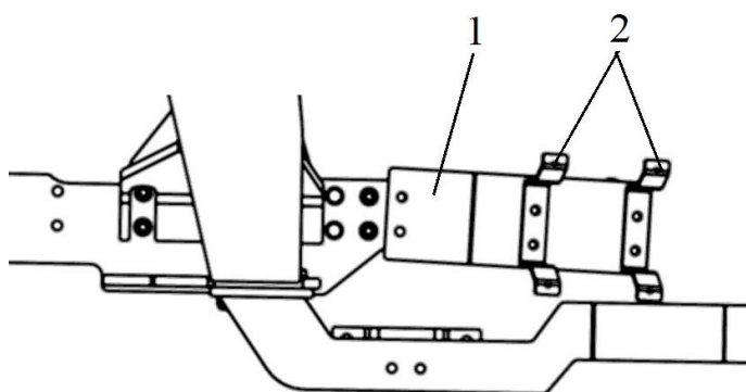
Рисунок 9Б- Установка ресивера КУН(TURS)-1500 на МТЗ 82.3 1- кронштейн КУН 1500.00.421; 2- скоба КУН 1500.00.422
