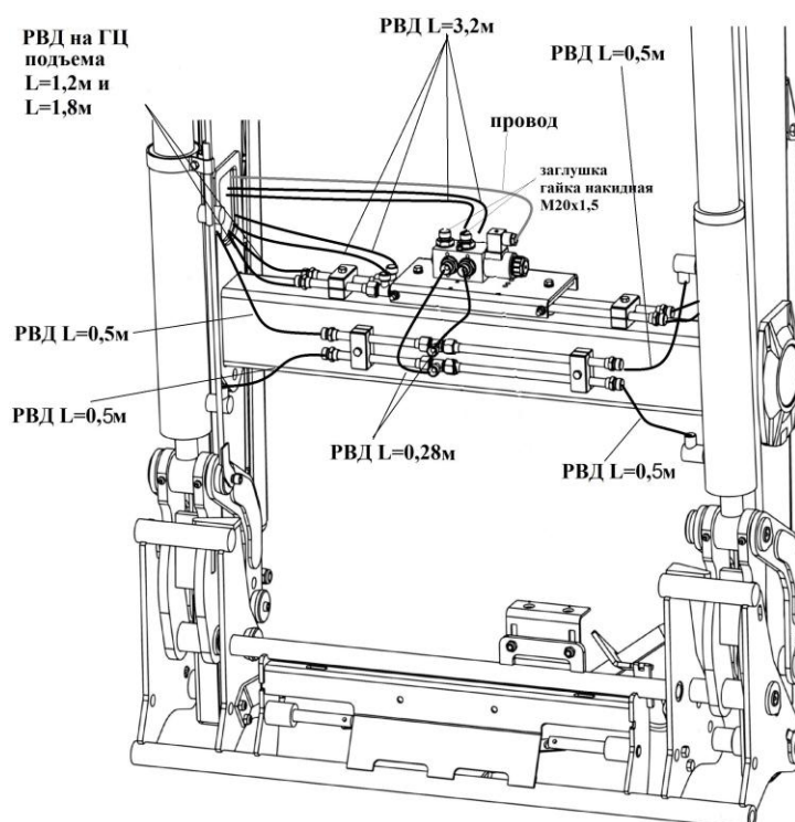
Рисунок 19А – Подсоединения РВД к дивертору для КУН(TURS)-1000-0Д
