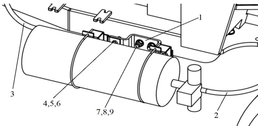
Рисунок 9А – Установка ресивера на КУН(TURS)-1500(МТЗ 1025.2, МТЗ 1025.3): 1-кронштейн КУН 2000.00.426-1025; 2-рукав 12,5х24-16В L=0,5 м; 3-рукав 12,5х24-16В L=0,8 м; 4-болт М12х40; 5-гайка М12; 6-шайба А.12.01; 7-болт М16х50; 8-гайка М16 DIN; 9-шайба А.16.01.
