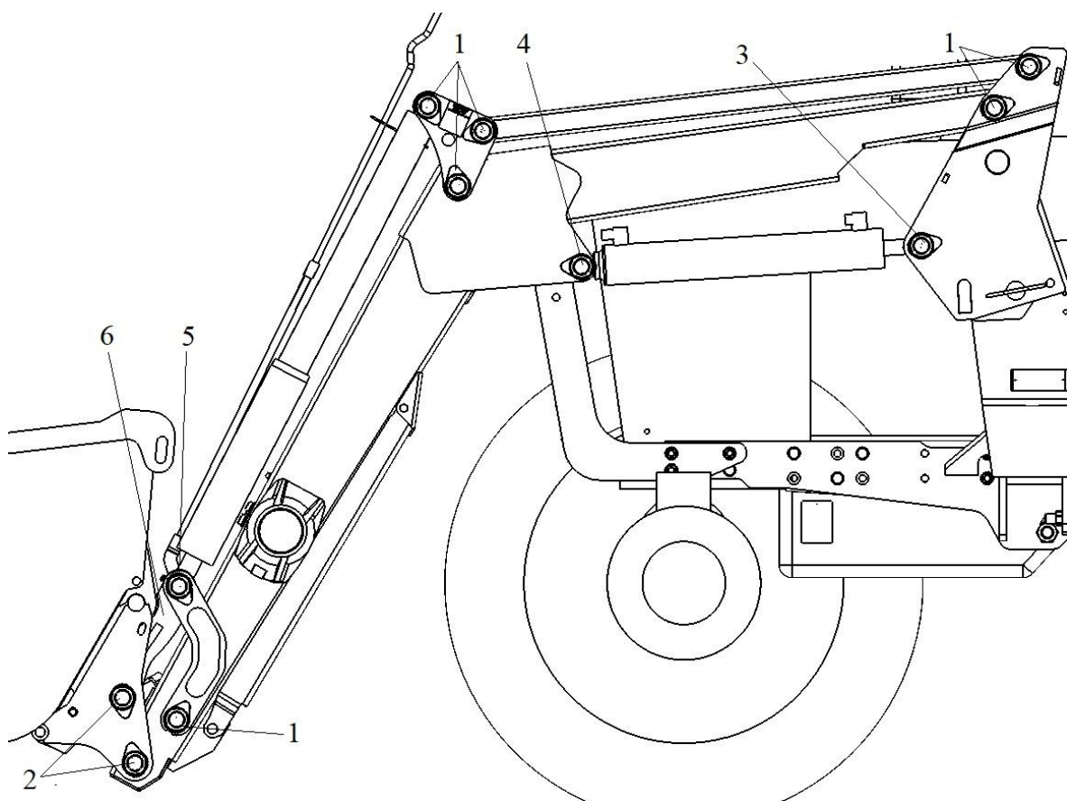
Схема расположения осей КУН(TURS)-1000
