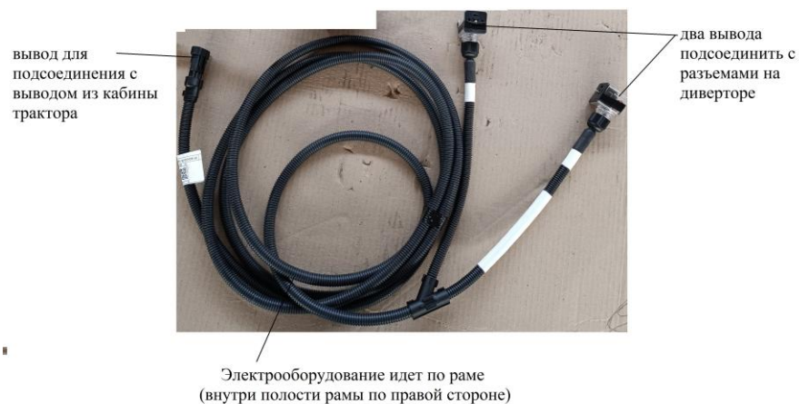
Рисунок 19В- Электрооборудование по раме для КУН-1500 и КУН-2000
