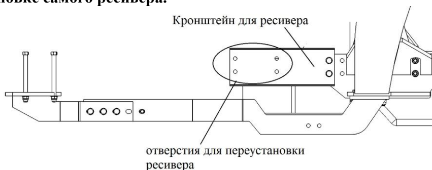
Рисунок 9 – Установка ресивера КУН(TURS)-2000
