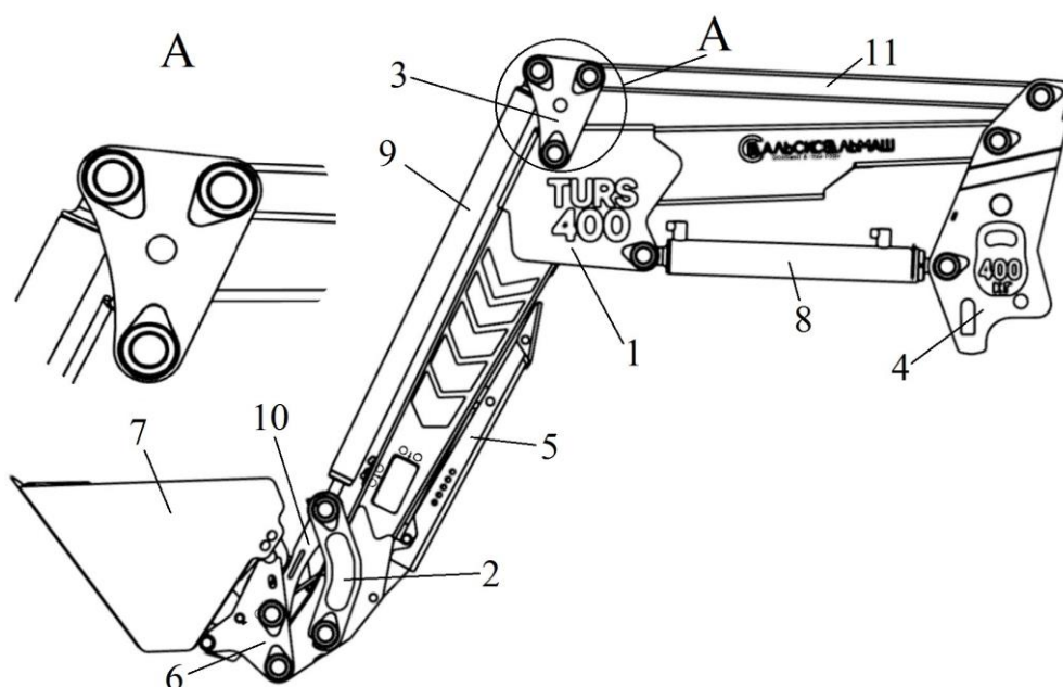
Рисунок 6 – Подъемное устройство:
