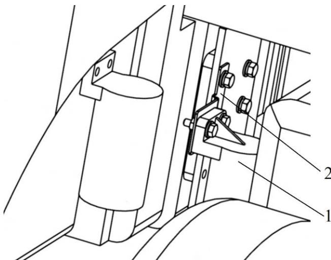
Рисунок 14 – Вид трактора слева: 1-кронштейн; 2-фильтр WBF1235.
