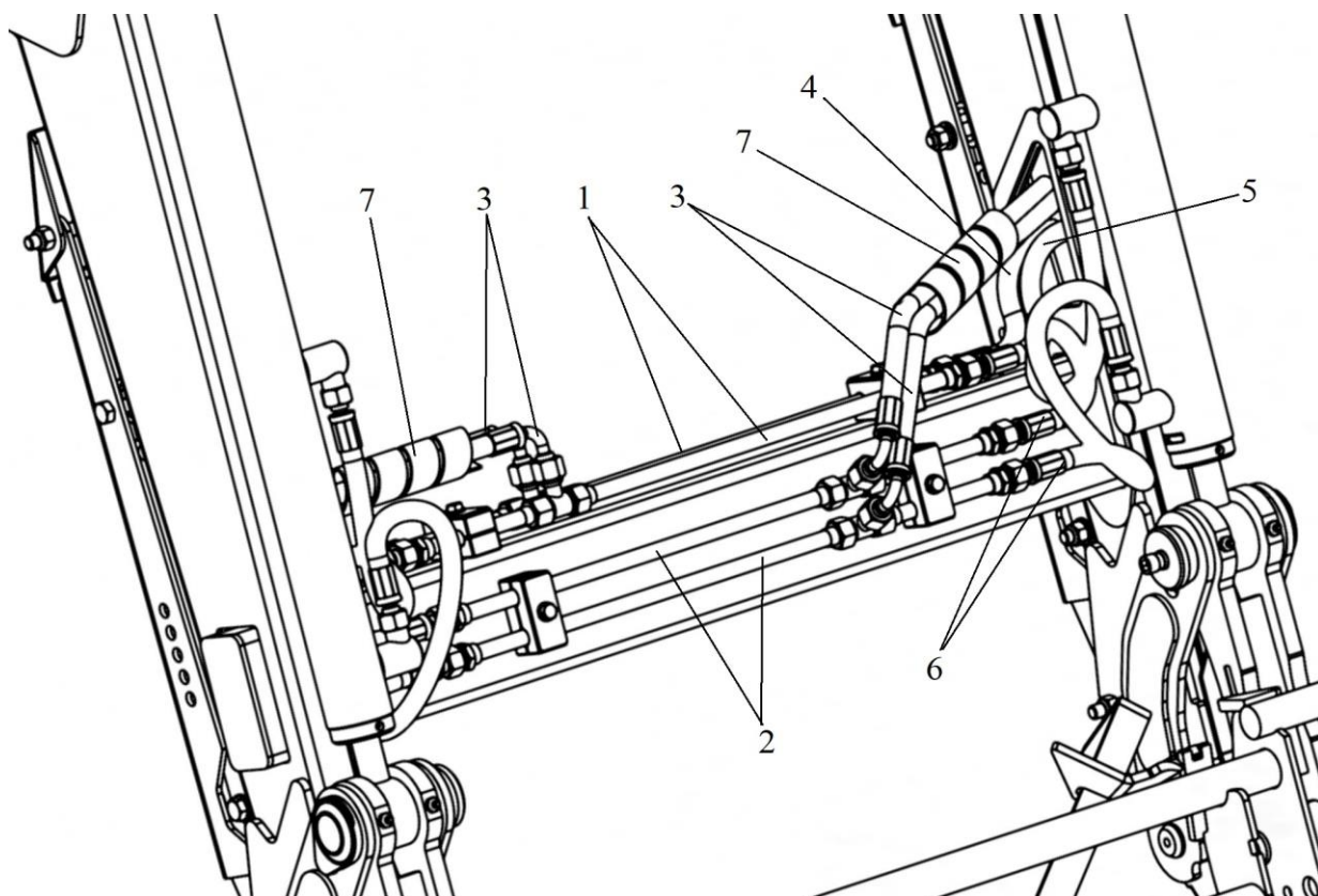
Рисунок 18 – Подсоединение ГЦ рабочих органов и ГЦ подъема к гидросистеме погрузчика:
