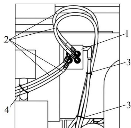
Рисунок 17 – Подсоединение гидросистемы погрузчика к гидросистеме трактора, вид сзади: 1-распределитель трактора; 2-РВД L=2,7 м; 3-хомут 3,6х200; 4-хомут 7,2х400.
