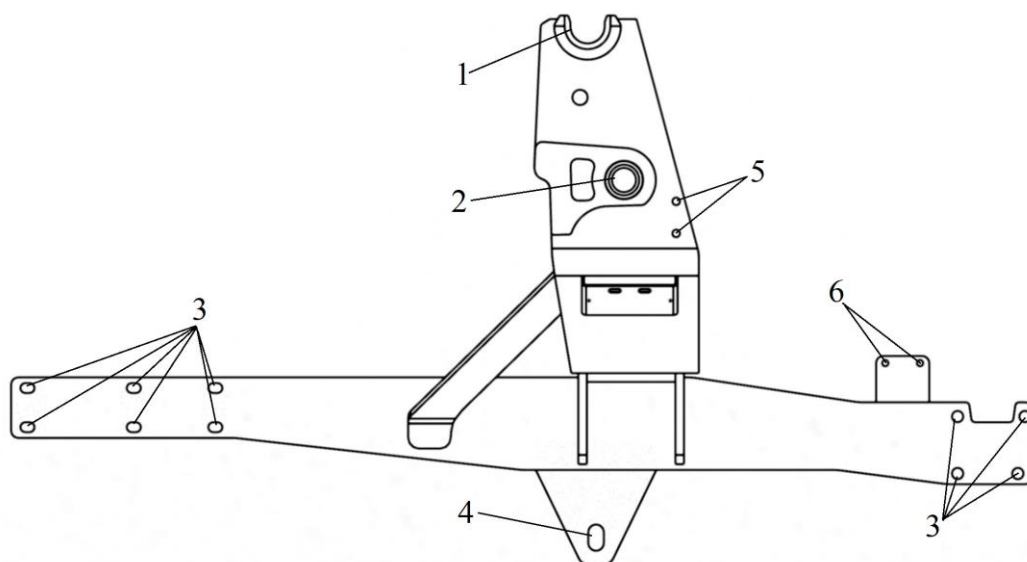
Рисунок 5 – Панель левая:
