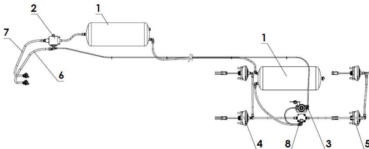
Rysunek 4.12. Schemat pneumatycznej instalacji hamulcowej dwuprzewodowej.
