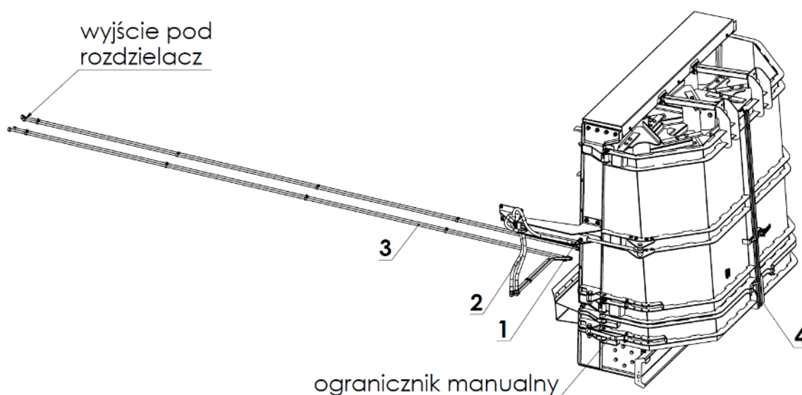
Rysunek 4.10. Budowa hydraulicznego otwierania deflektorów
