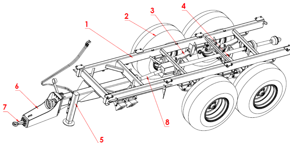
Rysunek 4.2. Podwozie rozrzutnika
