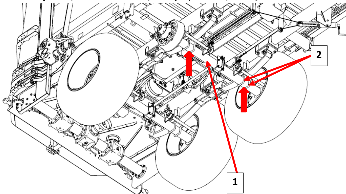
Rysunek 6.1. Punkt podparcia podnośnika
