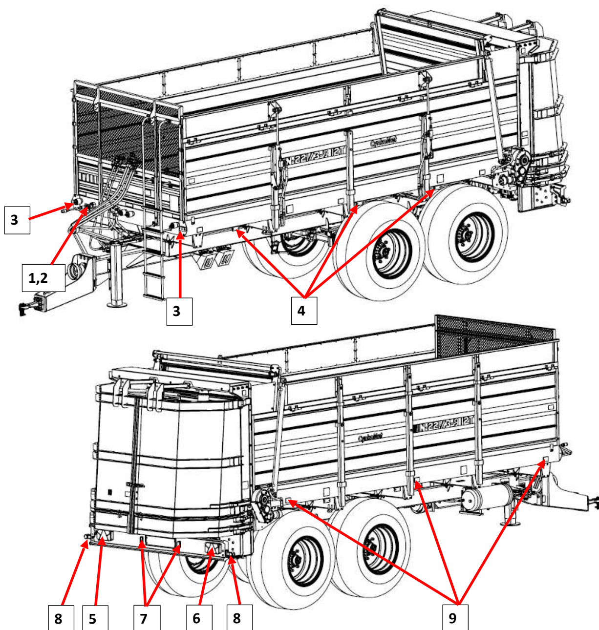
Rysunek 4.17. Schemat układu oświetlenia i sygnalizacji
