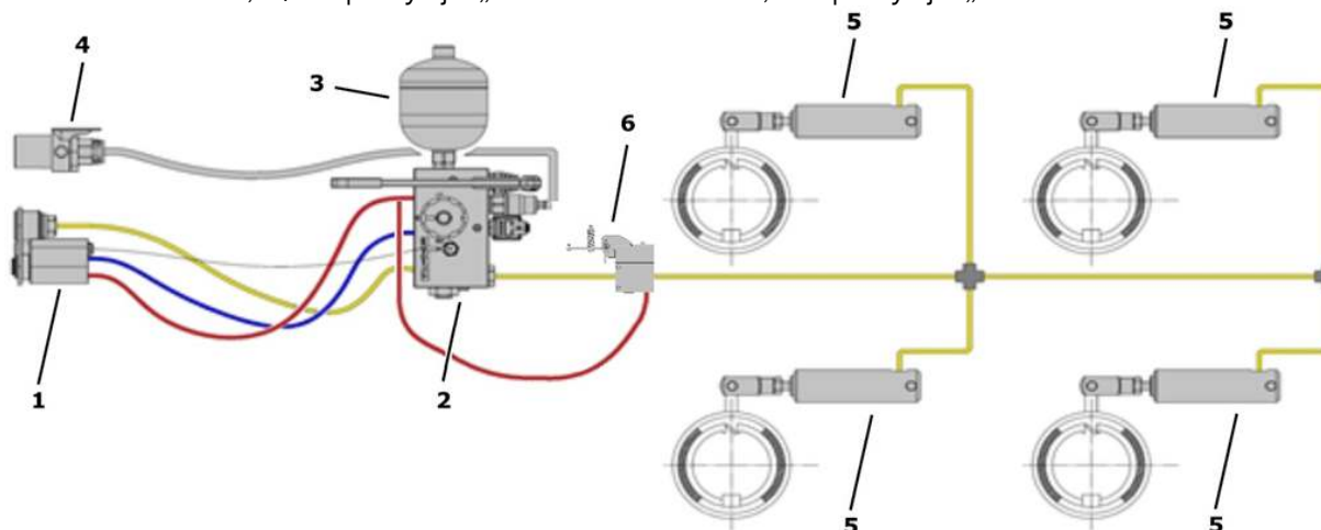
Rysunek 4.14. Schemat hydraulicznej instalacji hamulcowej.
