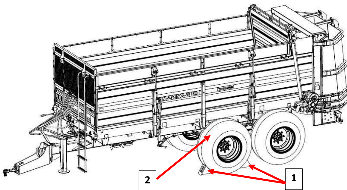
Rysunek 3.3. Sposób ustawiania klinów.
