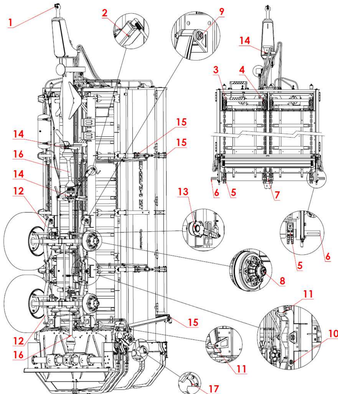
Rysunek 6.8. Rozmieszczenie punktów smarowania
