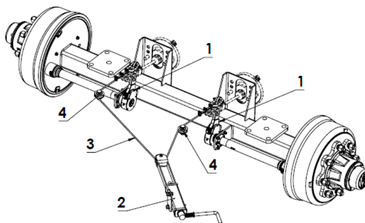
Rysunek 4.15 Hamulec postojowy
