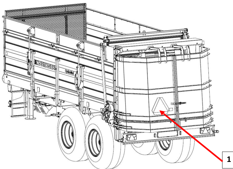
Rysunek 3.2. Miejsce umieszczenia tablicy wyróżniającej pojazdy wolno poruszające się.
