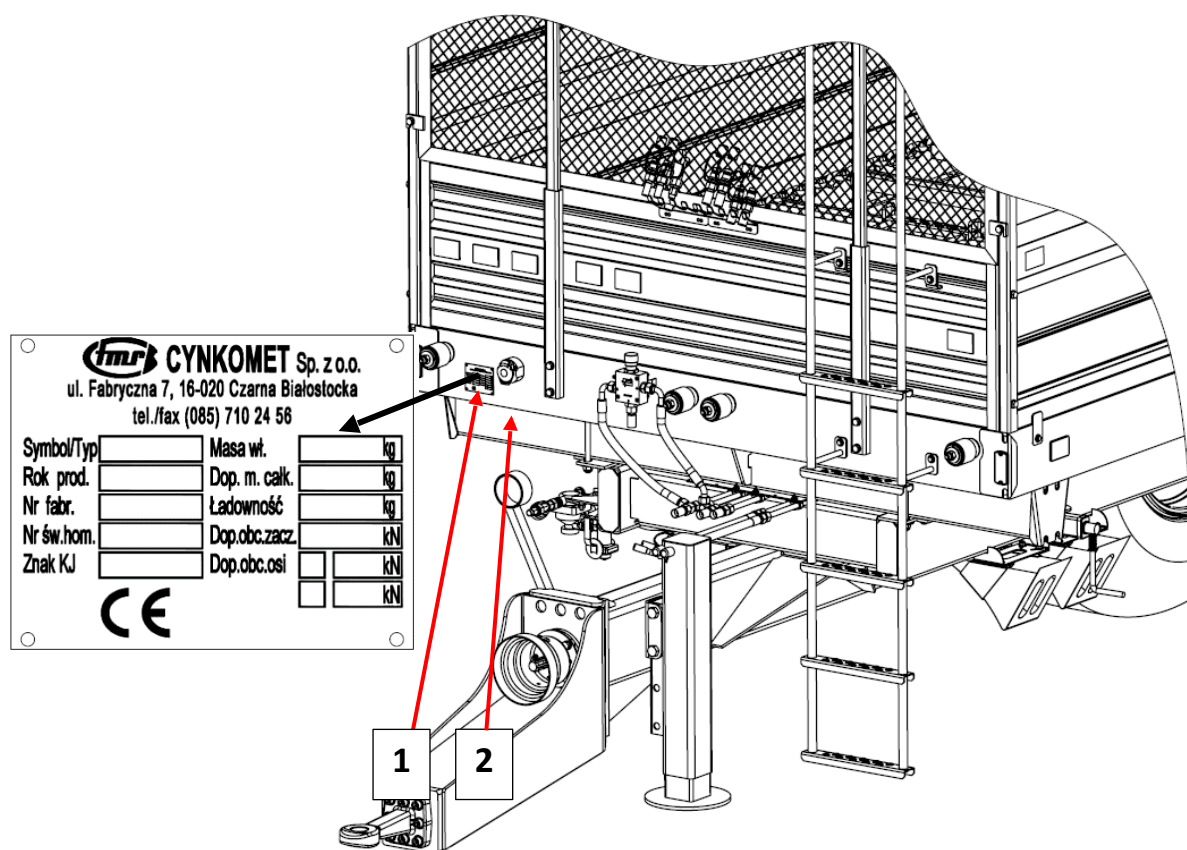
Rysunek 1.1. Miejsce umieszczenia tabliczki znamionowej i wybicia numeru fabrycznego, oraz wzór tabliczki znamionowej (homologacja PL)
