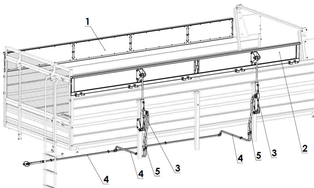
Rysunek 4.8. Budowa nadstaw 350
