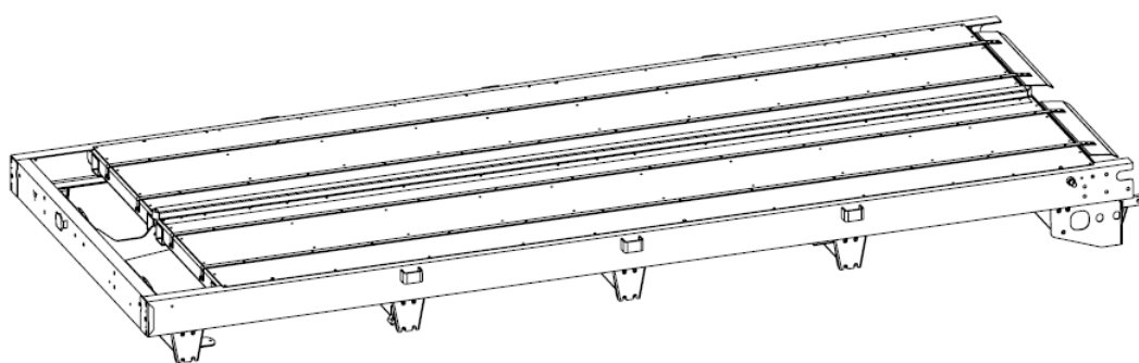
Rysunek 4.3 rama górna rozrzutnika
