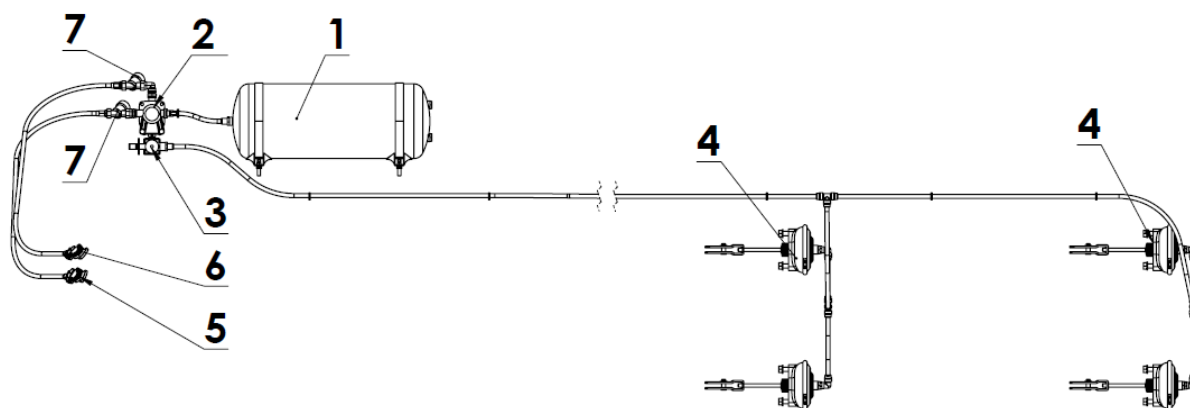
Rysunek 4.11. Schemat pneumatycznej instalacji hamulcowej dwuprzewodowej.
