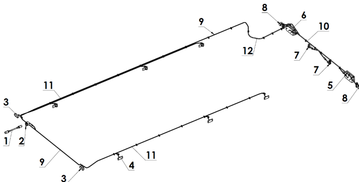
Rysunek 4.16. Schemat instalacji elektrycznej rozrzutnika.
