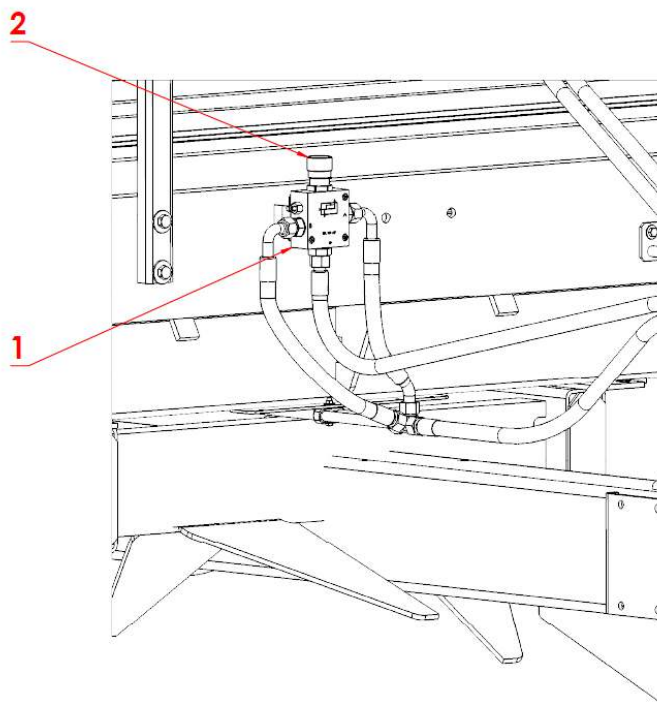
Rysunek 4.19. Regulacja prędkości przesuwu przenośnika podłogowego
