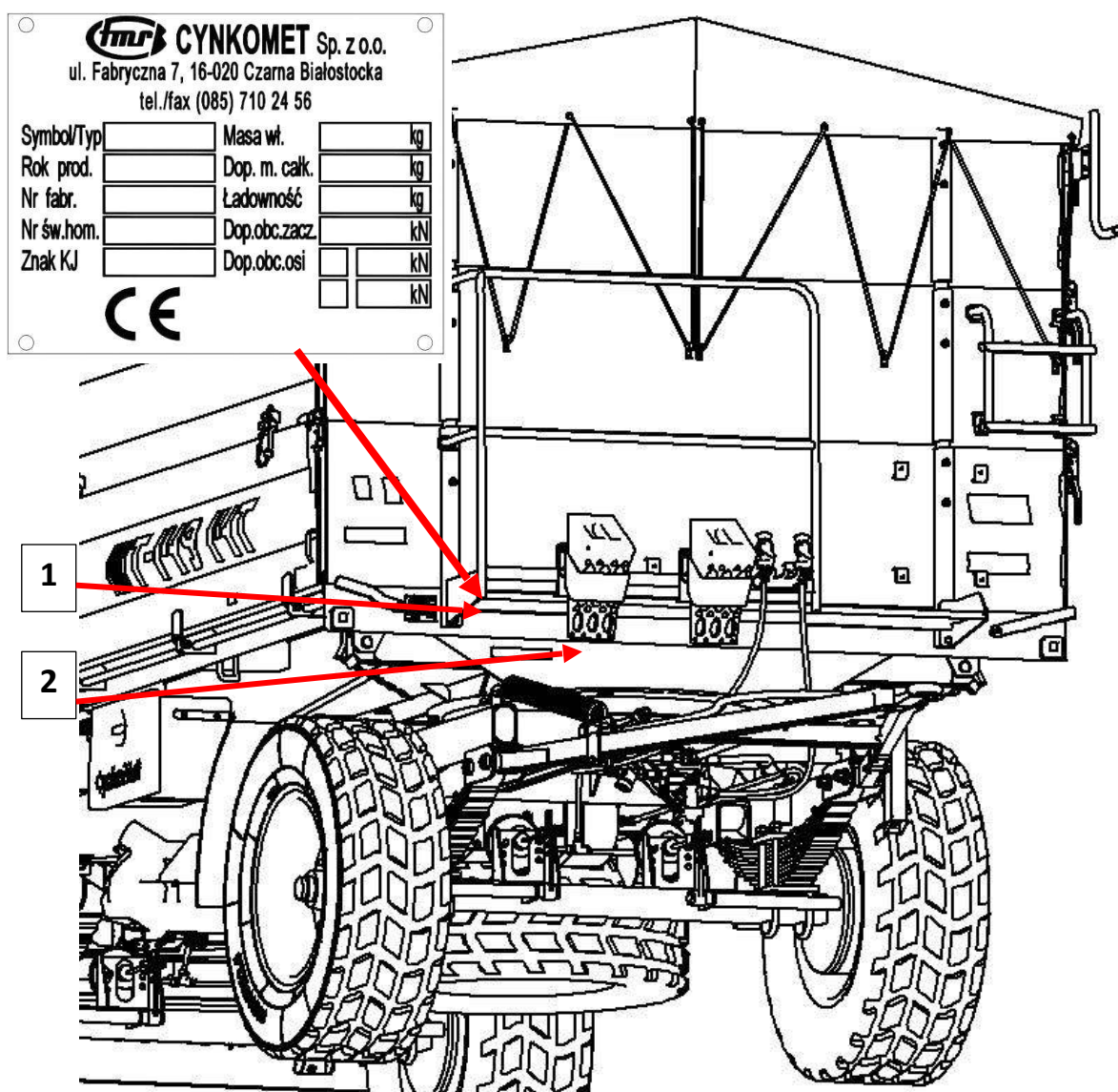
Rysunek 1. Miejsce umieszczenia tabliczki znamionowej i wybicia numeru fabrycznego, oraz wzór tabliczki znamionowej (homologacja PL)
