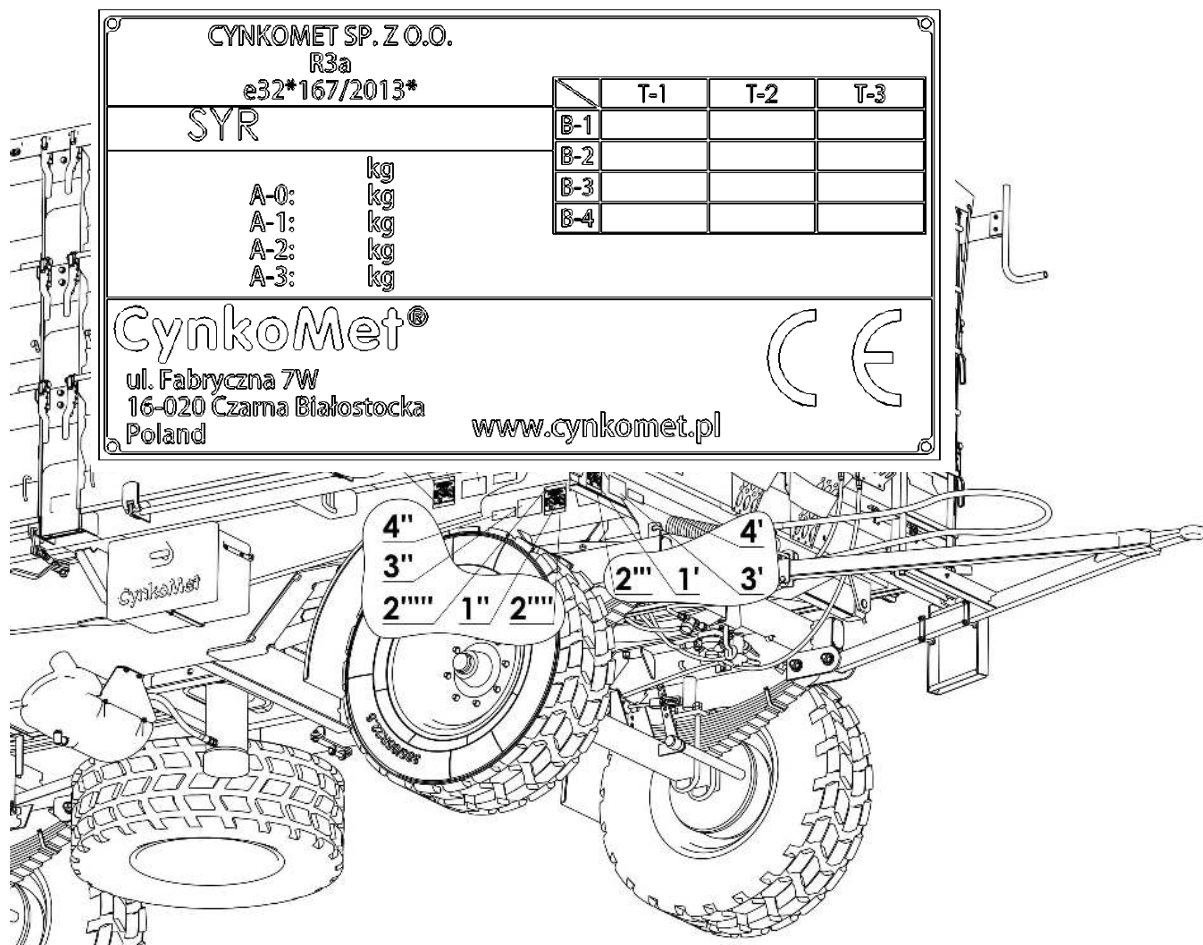
Rysunek 2. Możliwe miejsce umieszczenia tabliczki znamionowej i wybicia numeru fabrycznego, oraz wzór tabliczki znamionowej (homologacja EU).
