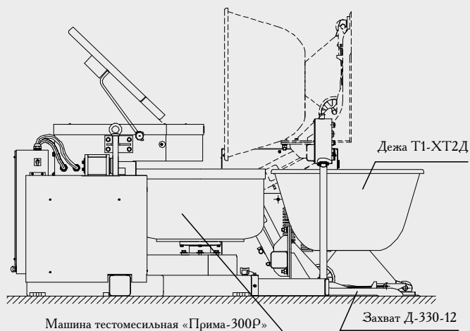
Опрокидывание дежи Т1-ХТ2Д с захватом Д-330-12 в составе машины тестомесильной «Прима-300Р»
