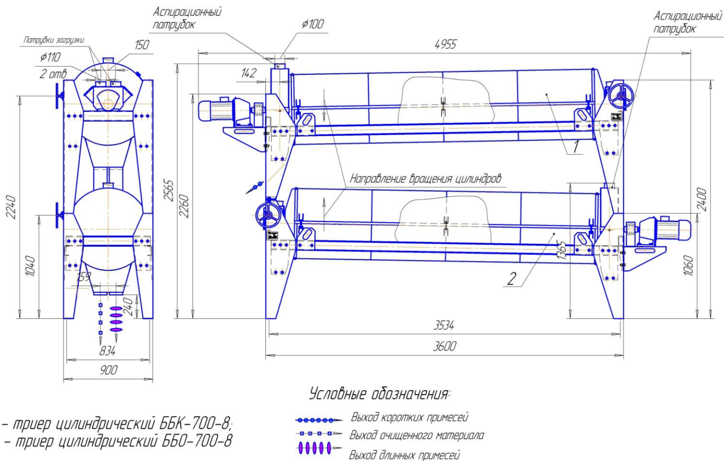
Рисунок 2-Габаритные, установочные и присоединительные размеры блока триерного P1-ББТ-700-8
