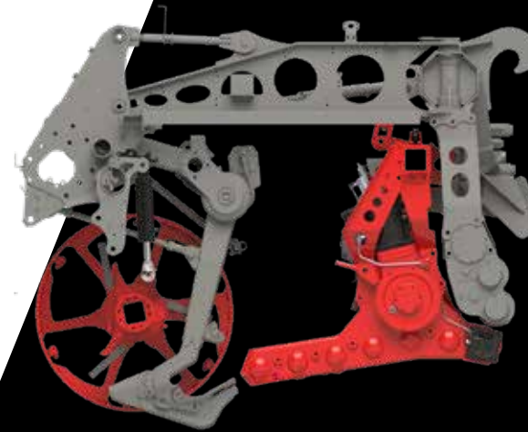
Zwangseinzugschwelle vorne für leichte Böden
