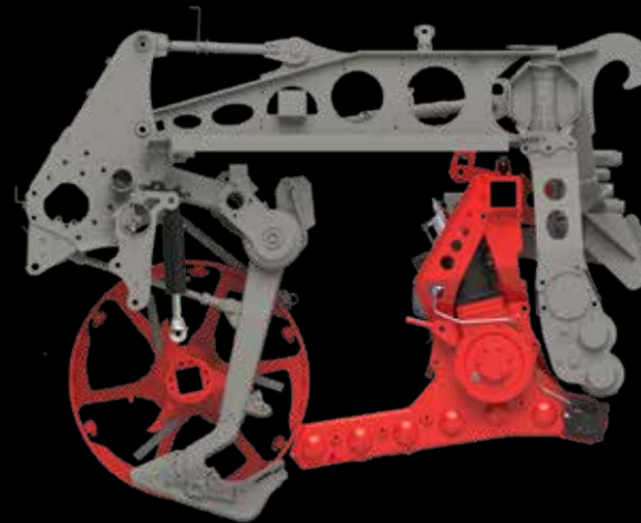
Zwangseinzugschwelle hinten für schwere Böden
