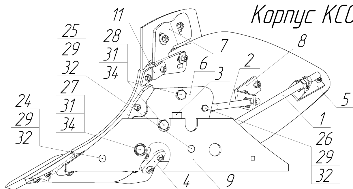
Корпус КСО-45 00.00.000-01
