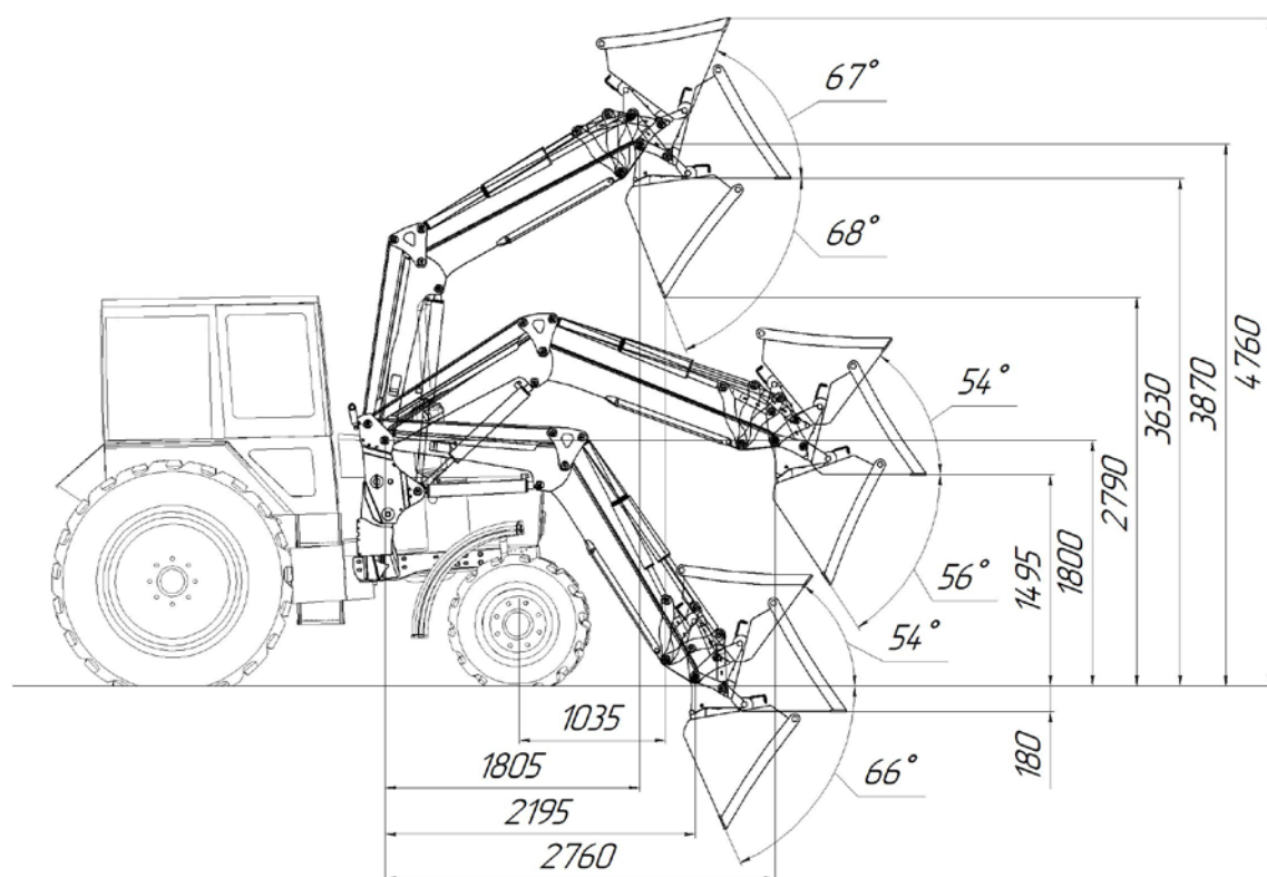
Рис. 1.7 – Габаритные размеры погрузчика Универсал VIP
