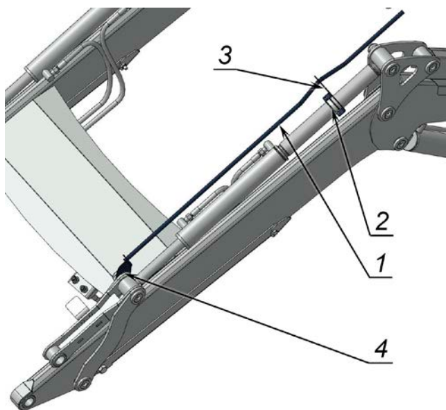
Рис. 1.23 – Указатель уровня ковша
