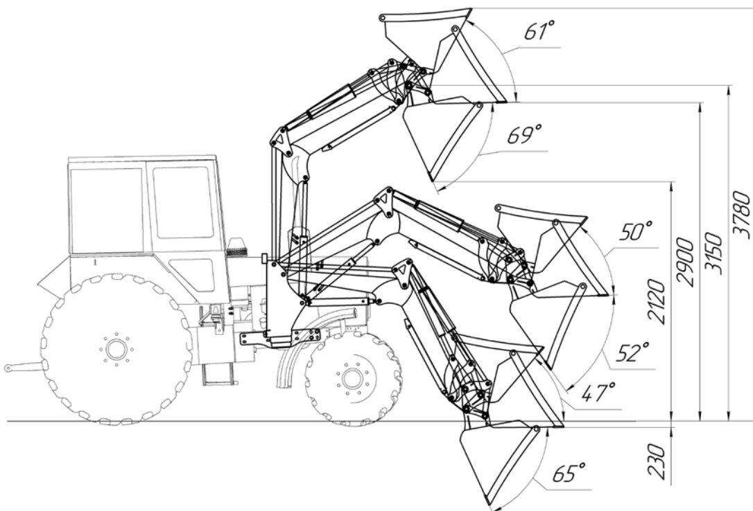
Рис. 1.2 – Габаритные размеры погрузчика Универсал Robust 650
