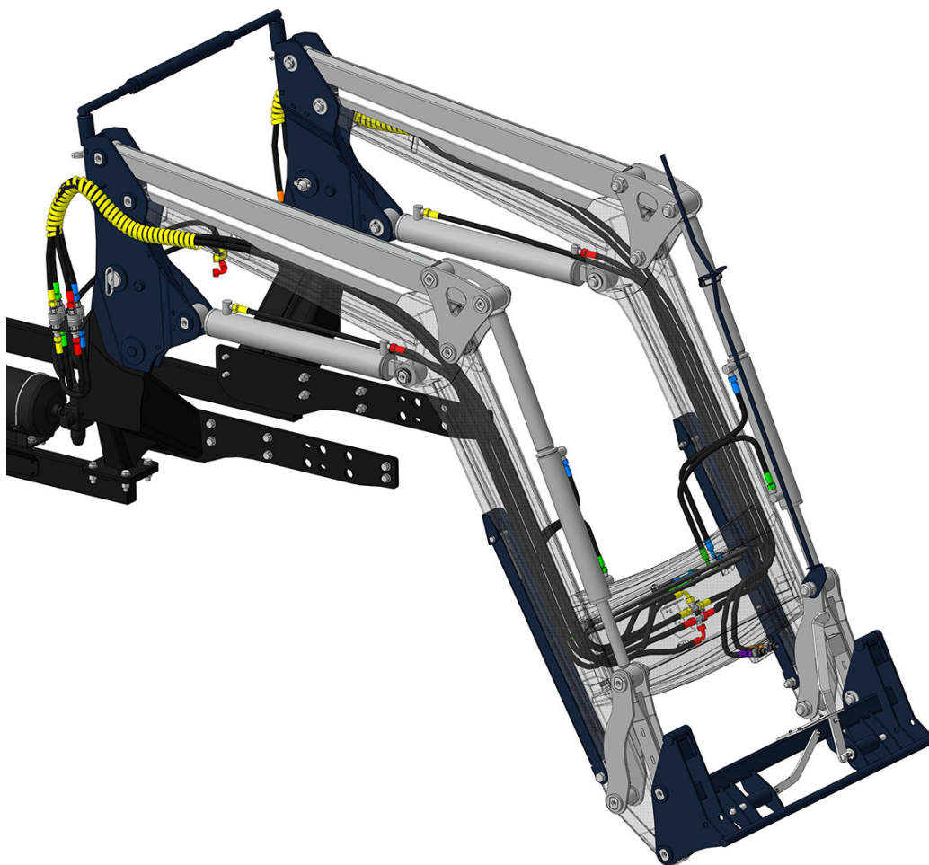
Рис. 1.27 – Гидросистема погрузчика
