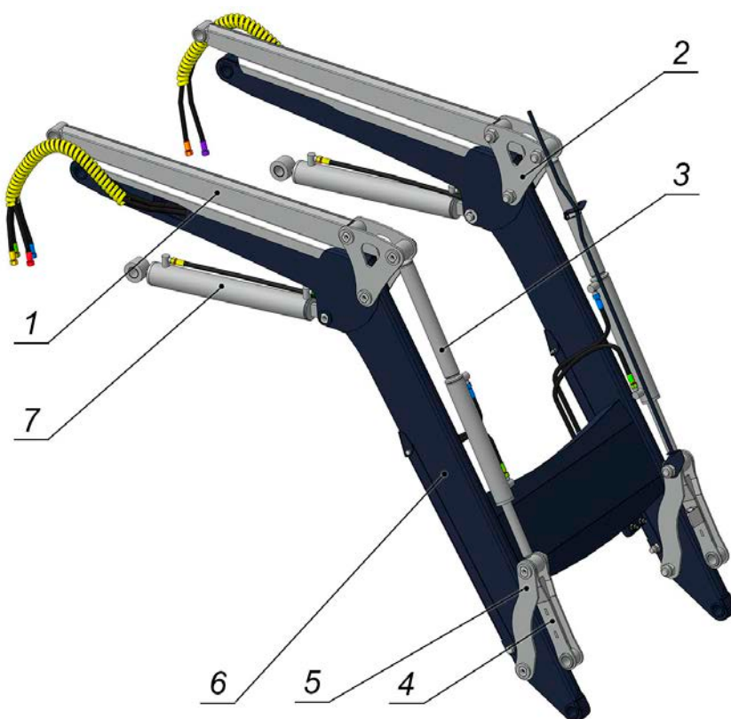
Рис. 1.21 – Стрела в сборе
