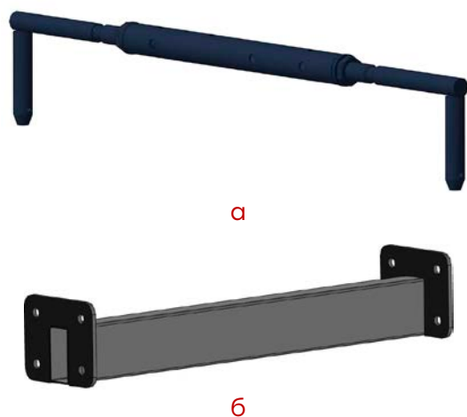
Рис. 1.15 – Распорка Универсал Premium: регулируемая (а), нерегулируемая нижняя (б)
