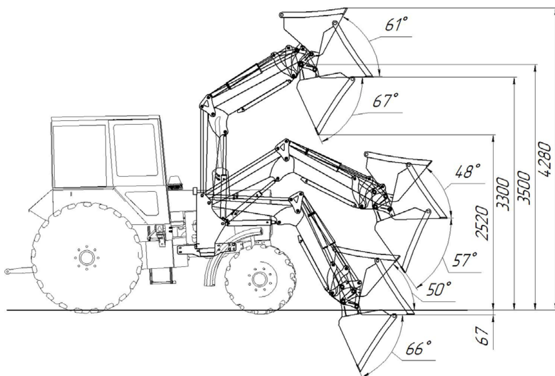
Рис. 1.3 – Габаритные размеры погрузчика Универсал Lite
