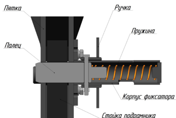
Рис. 1.19 – Полуавтоматический механизм фиксации
