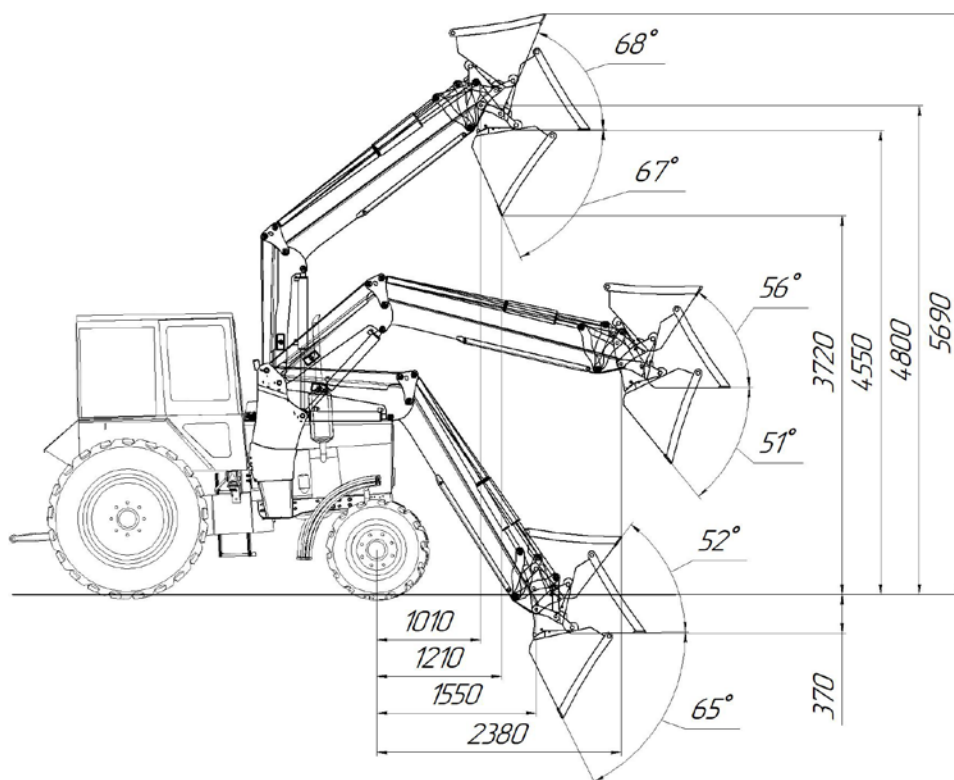
Рис. 1.9 – Габаритные размеры погрузчика Универсал 4,5
