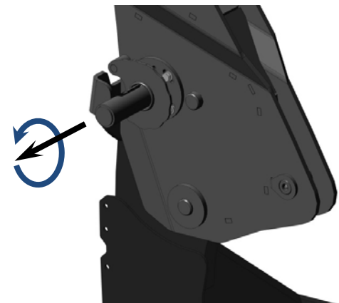
Рис. 2.5 – Раскрепление пятки Универсал Premium
