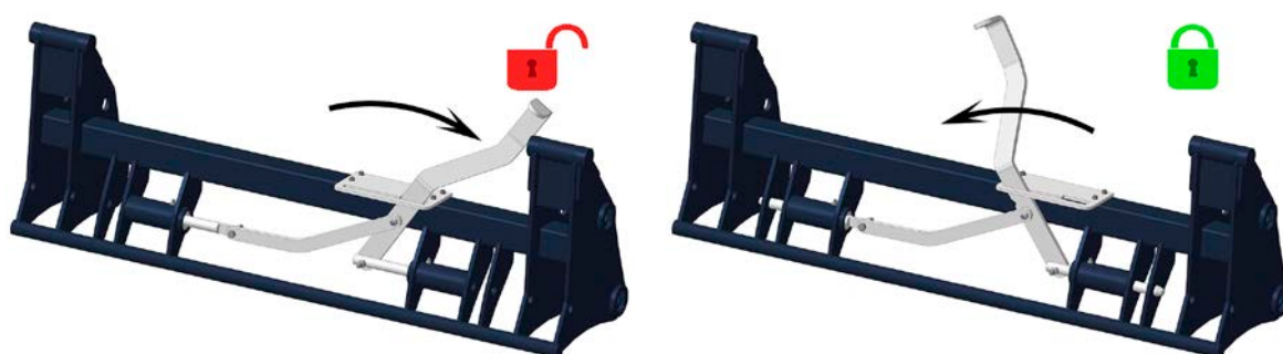
Рис. 1.25 – Подвеска Универсал 400, Универсал Robust 650, Универсал Standard, Универсал Robust, Универсал VIP, Универсал Premium, Универсал 4,5
