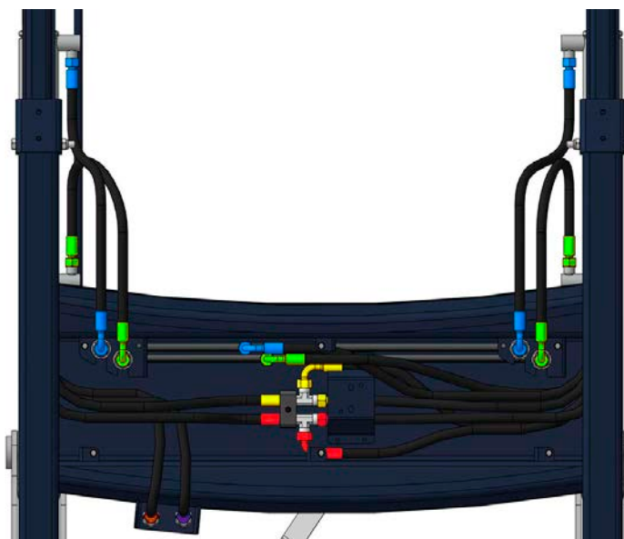
Рис. 1.28 – Разводка гидросистемы в поперечной балке
