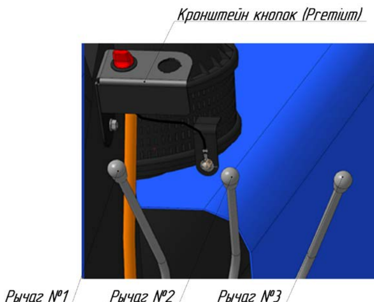
Рис. 1.29 – Органы управления погрузчиком Универсал
