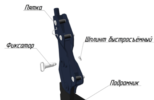
Рис. 1.18 – Ручной механизм фиксации
