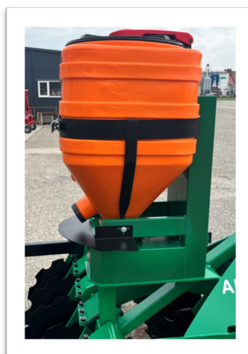
Halterung + elektrischer Spreizer
