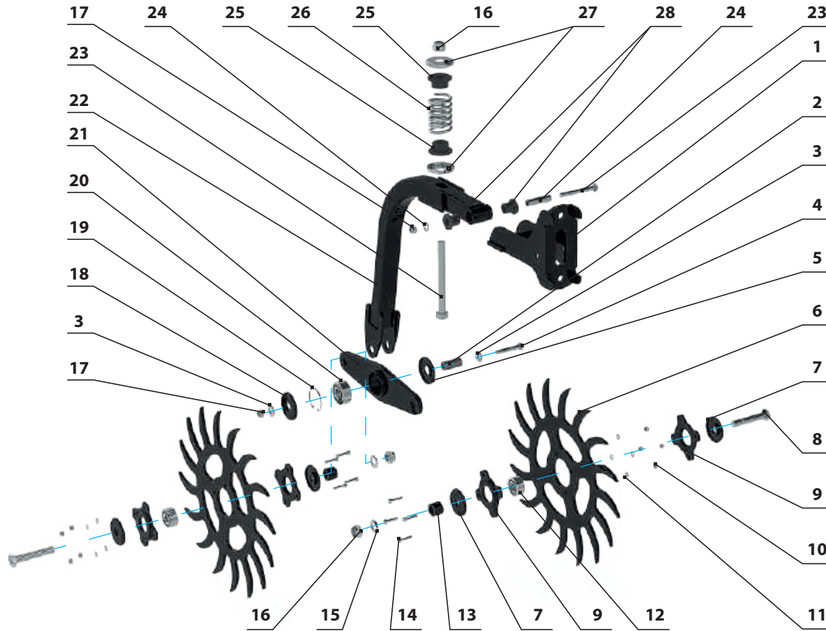
РОБОЧИЙ ОРГАН РОТАЦІЙНОЇ БОРОНИ
