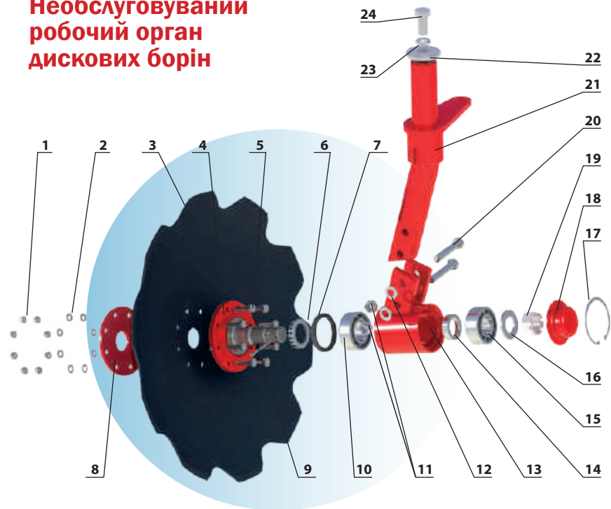
СТІЙКА З ДИСКОМ РКAB-174.04.850-05;06
