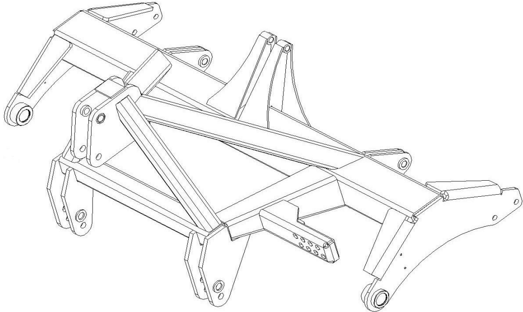
АДК-4.01.000 Рама
