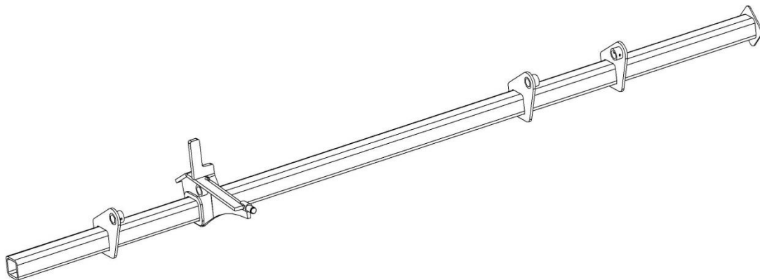
АДК-4.02.000 Балка
