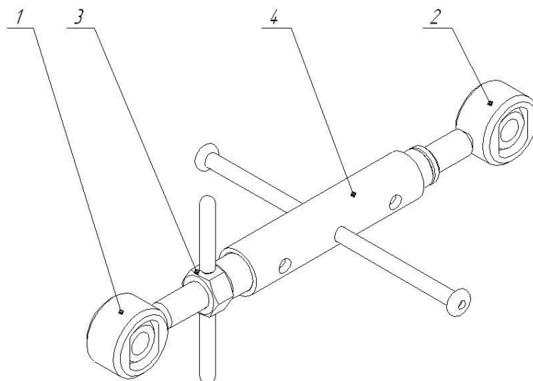
КДК-4.06.000 Талреп
