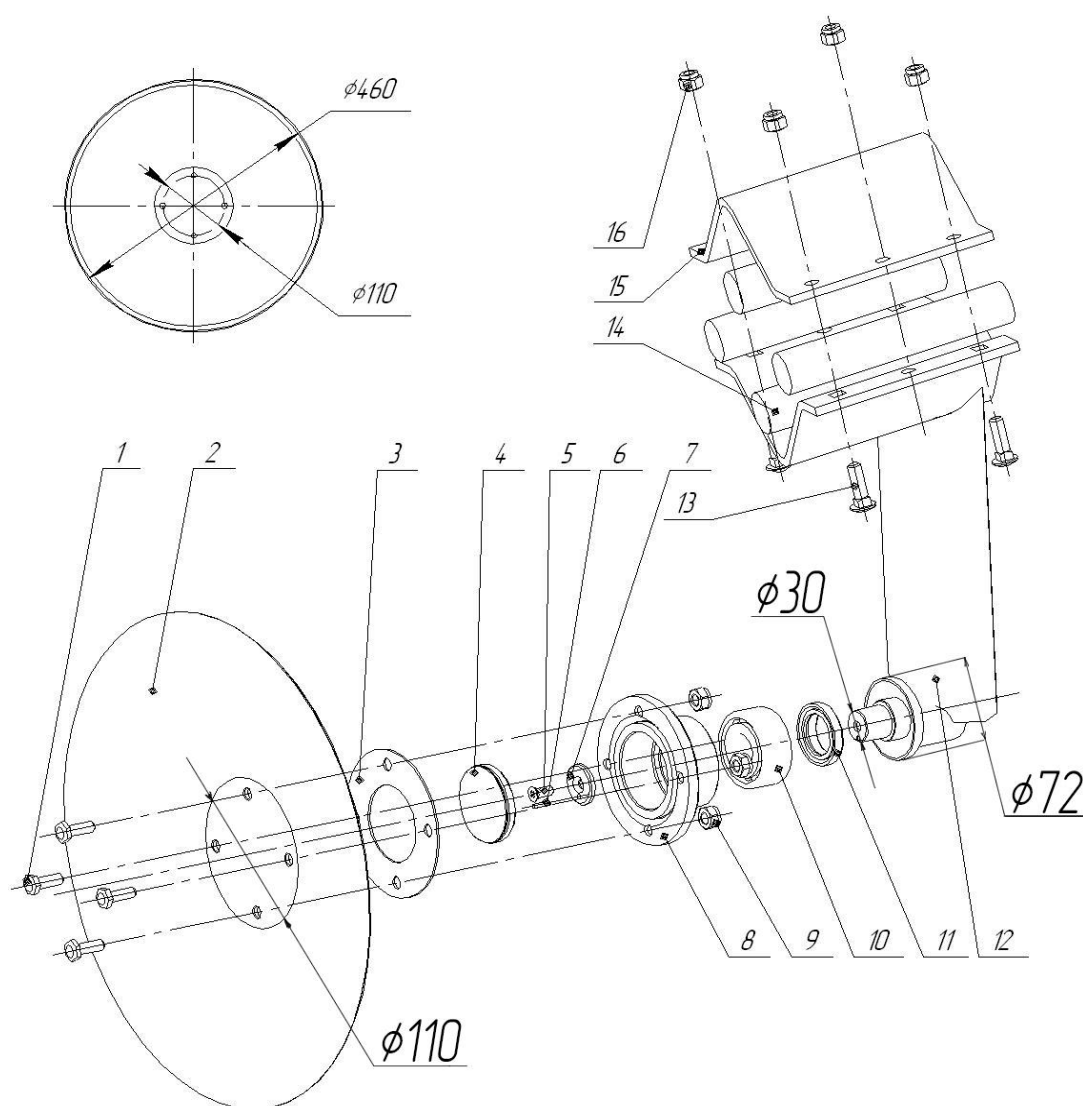
КДК-4.03.000 Стойка дисковая правая
