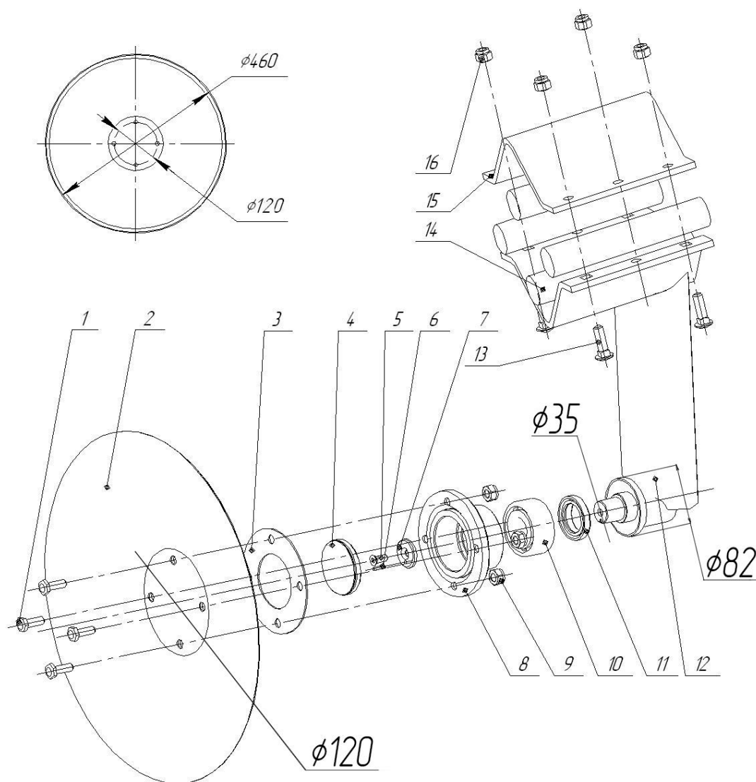
КДК-4.14.000 Стойка дисковая правая
