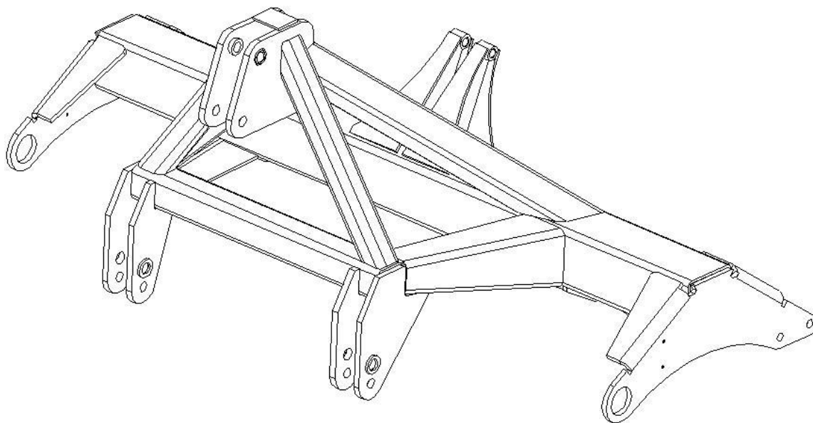
КДК-4.40.000 Рама
