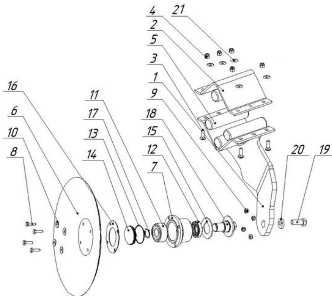
КДК-4.60.000 Стойка дисковая
