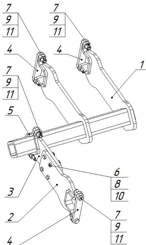
КДК-4.00.500 Стяжка
