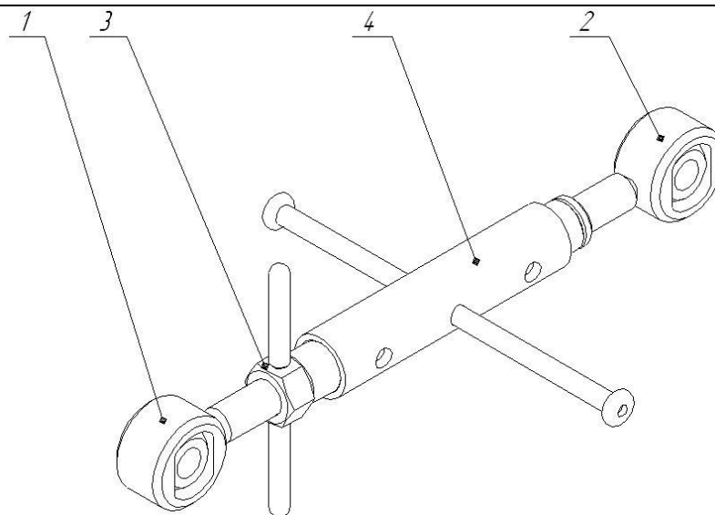
КДК-4.06.000 Талреп
