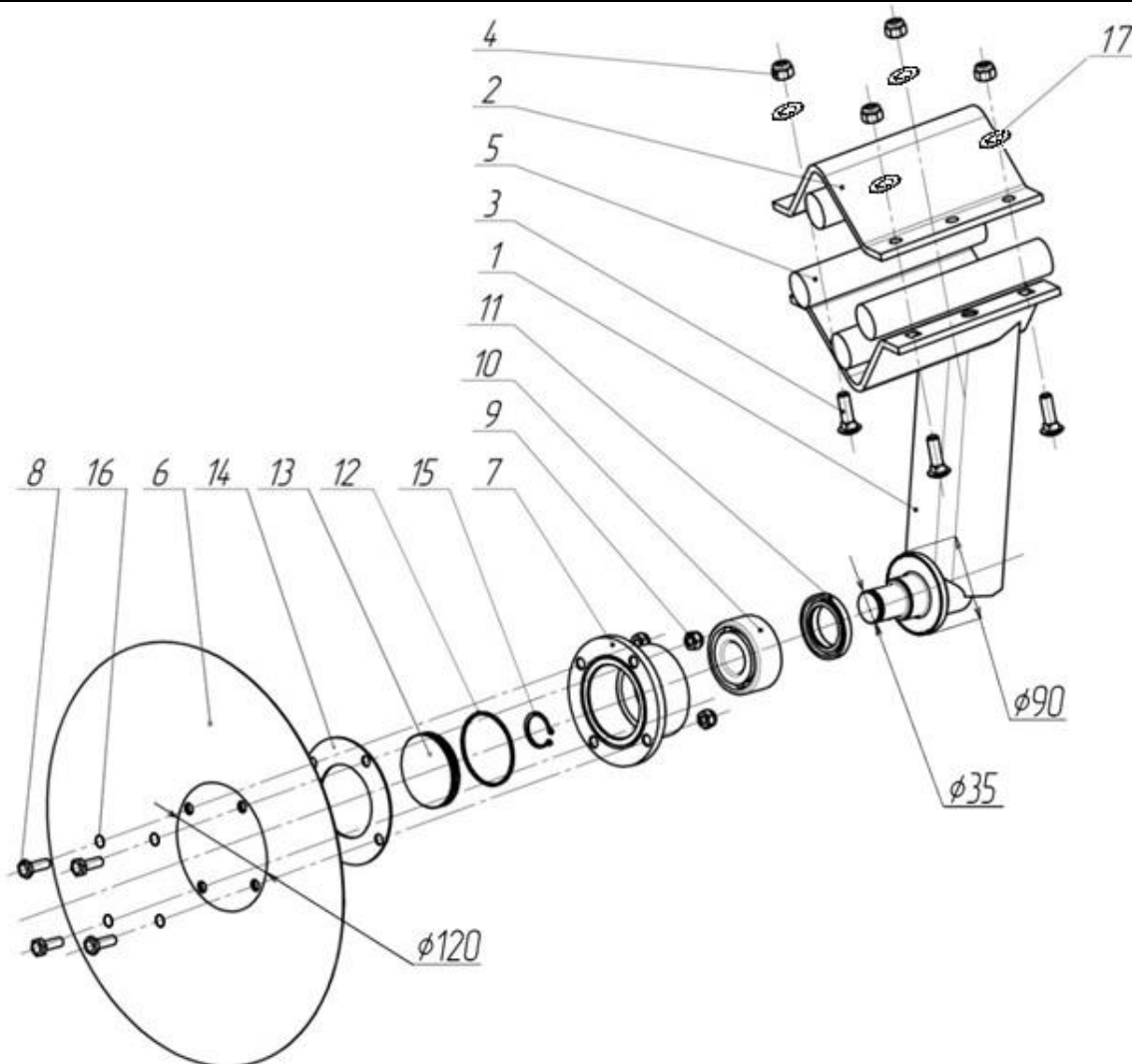
КДК-4.18.000 Стойка дисковая правая
