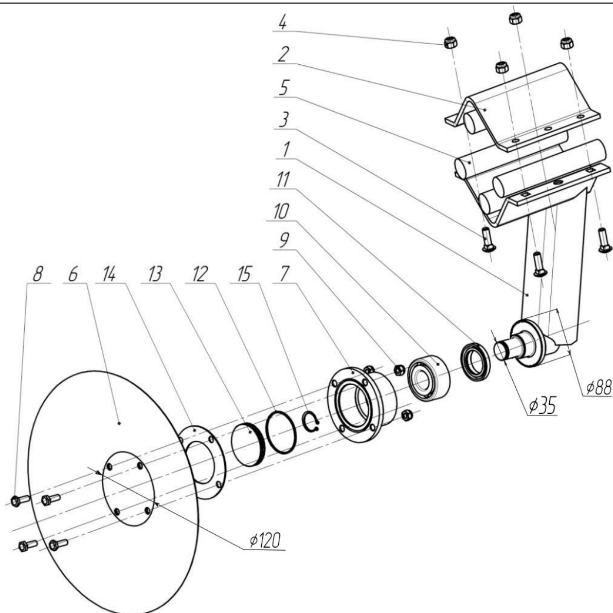
КДК-4.16.000 Стойка дисковая правая
