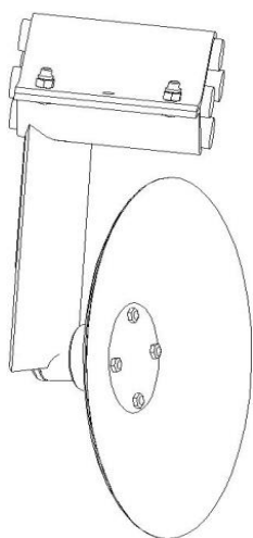
Рис.10.10.1 - КДК-4.18.000-01 Стойка дисковая левая
