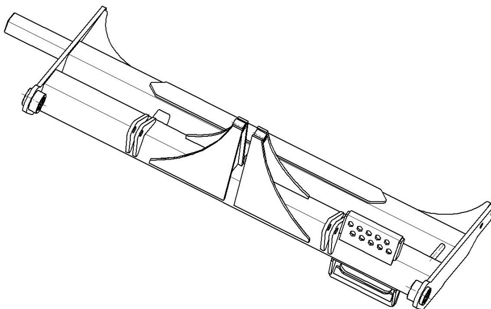
Рис.10.6.1 – КДК-6.03.100-01 Рама
