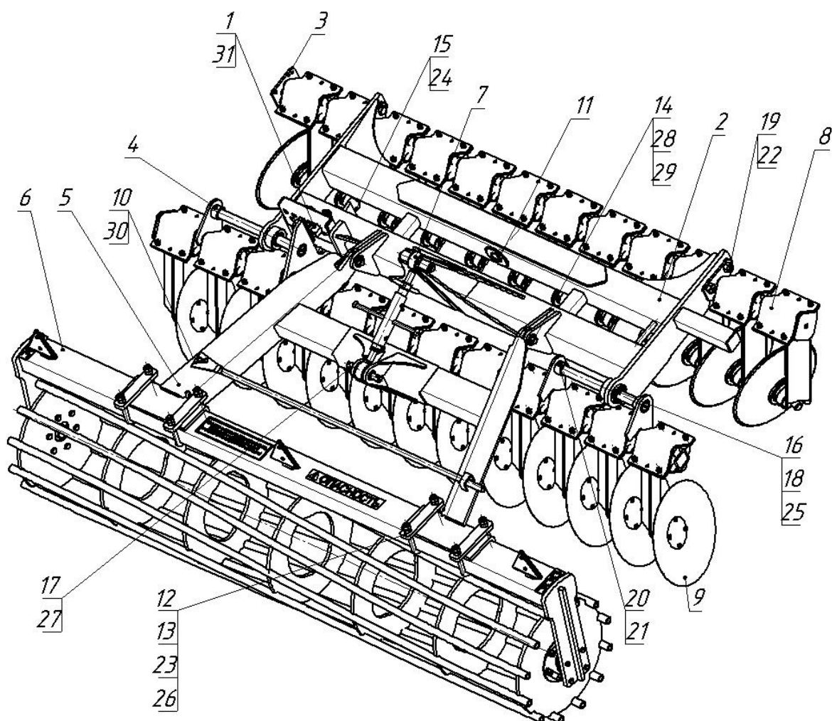
Рис.10 – КДК-6.03.000 Секция культиваторная (с трубчатым прикатчиком)
