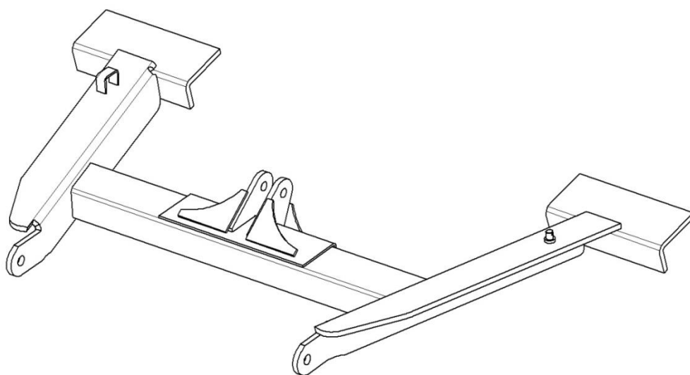
Рис.10.9 – КДК-6.03.400 Кронштейн прикатчика
