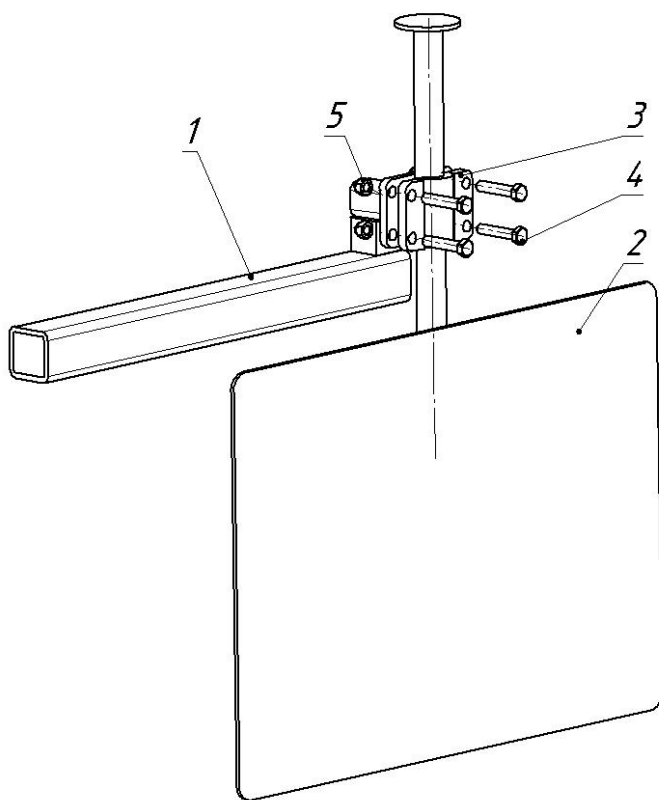
Рис.7 – КДК-6.00.400 Отражатель
