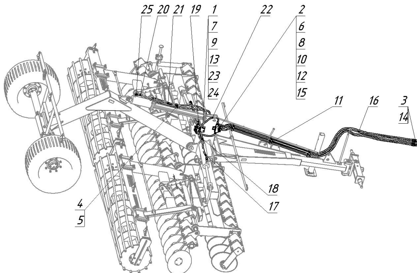
Рис.12- КДК-6.05.000 Гидрооборудование
