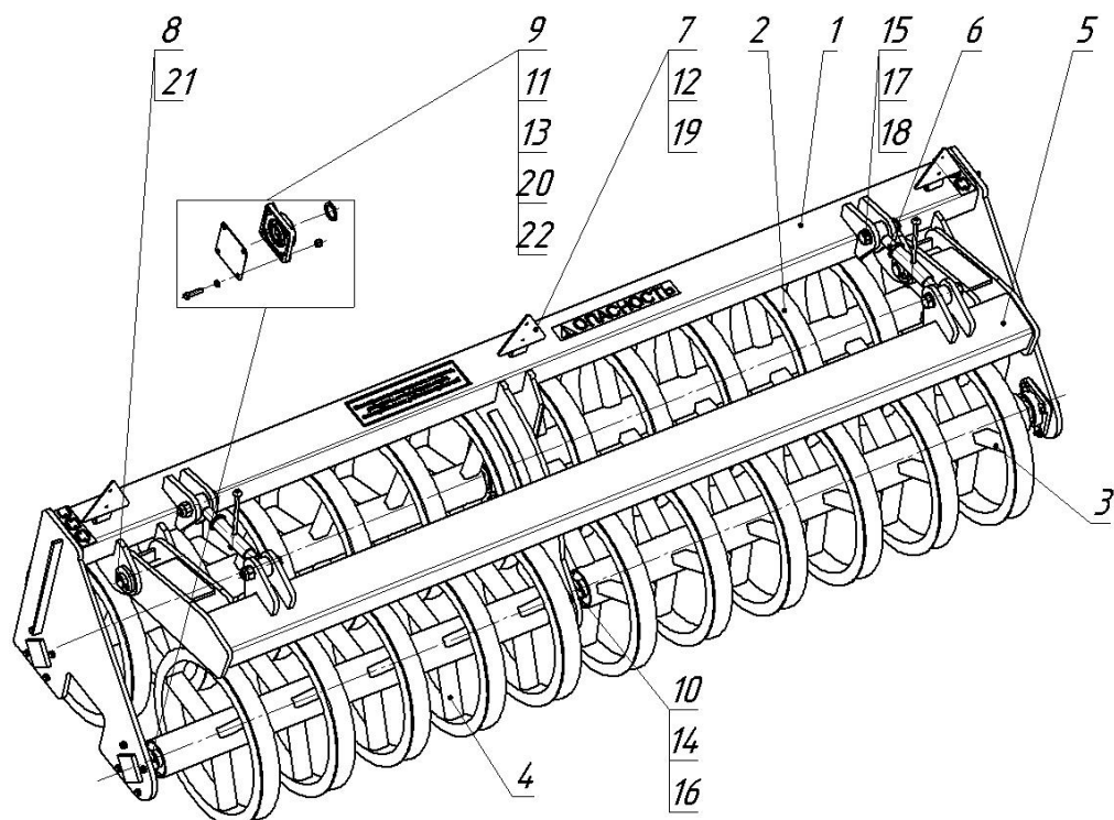
Рис.10.14 - КДК-3.50.000 Прикатчик
