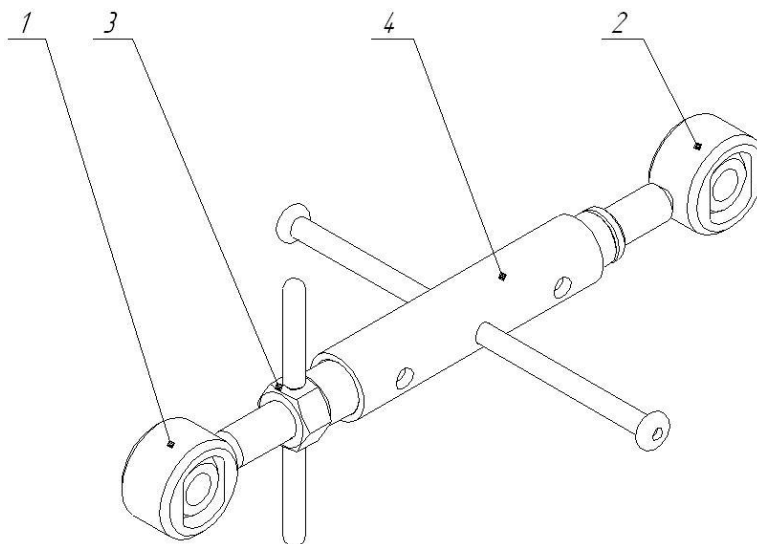
Рис.10.11 - КДК-4.06.000 Талреп
