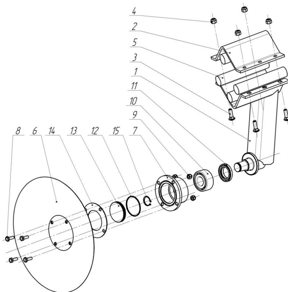
Рис.10.10 - КДК-4.18.000 Стойка дисковая правая
