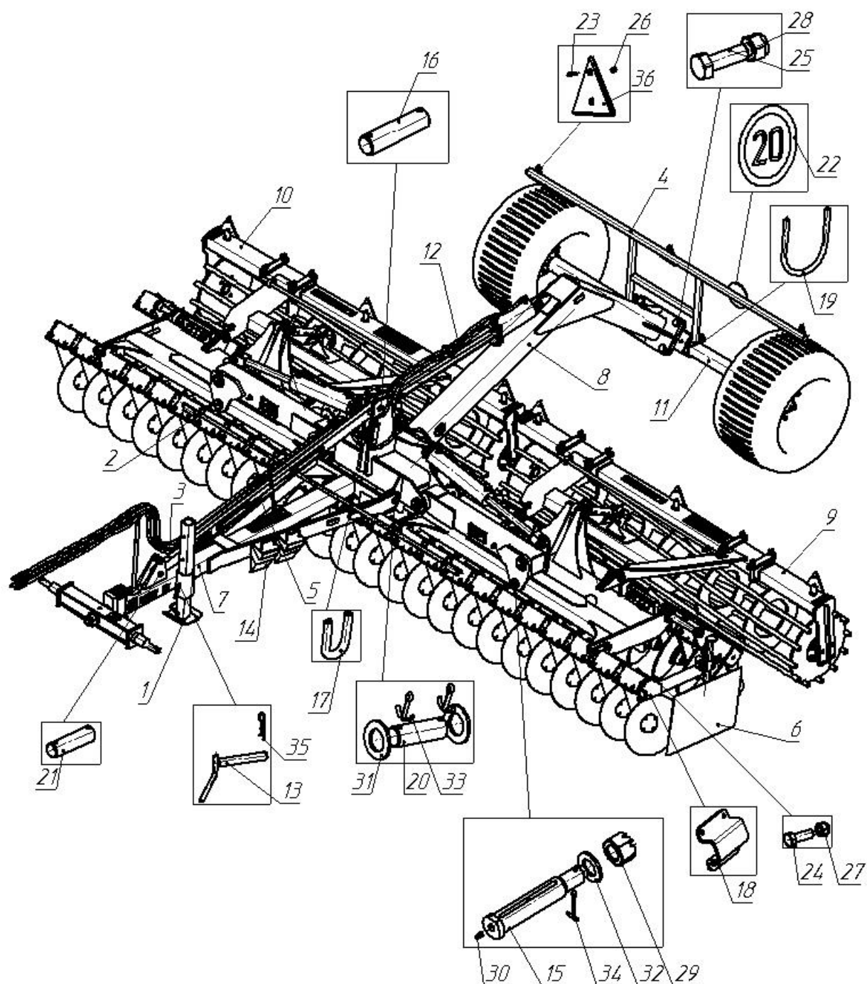
Рис.1 – КДК-6.00.000 СБ (с трубчатыми прикатчиками)
