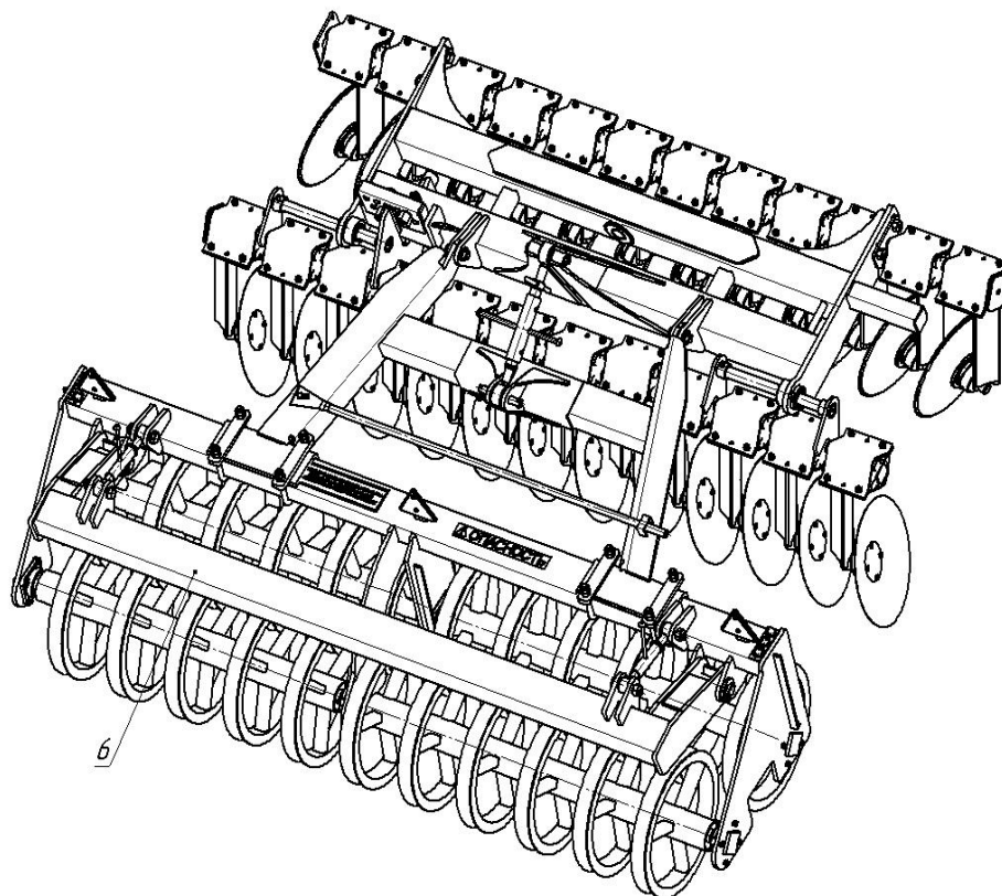
Рис.10.4 - КДК-6.03.000-04 СБ (с П-образным прикатчиком) (см. КДК-6.03.000 СБ)
