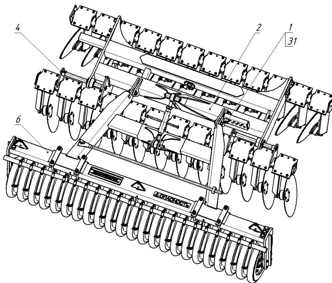
Рис.10.3 - КДК-6.03.000-03 СБ (с резиновым прикатчиком) (см. КДК-6.03.000 СБ)
