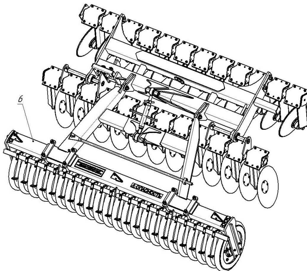
Рис.10.2 - КДК-6.03.000-02 СБ (с резиновым прикатчиком) (см. КДК-6.03.000 СБ)
