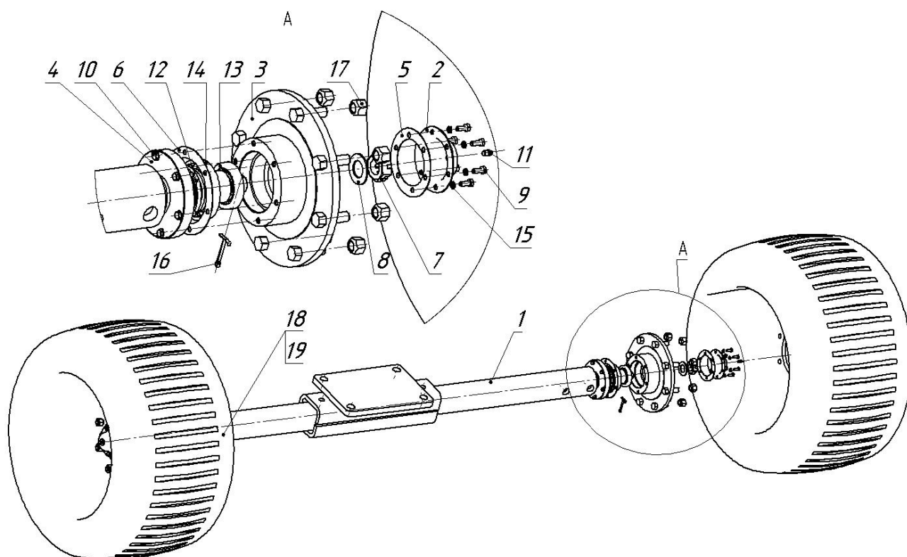
Рис.11- КДК-6.04.000 Шасси
