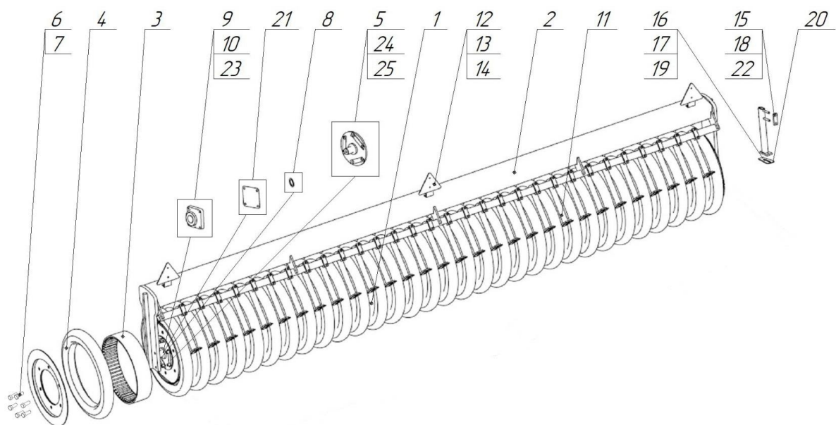
Рис.10.13 - КДК-3.36.000 Прикатчик
