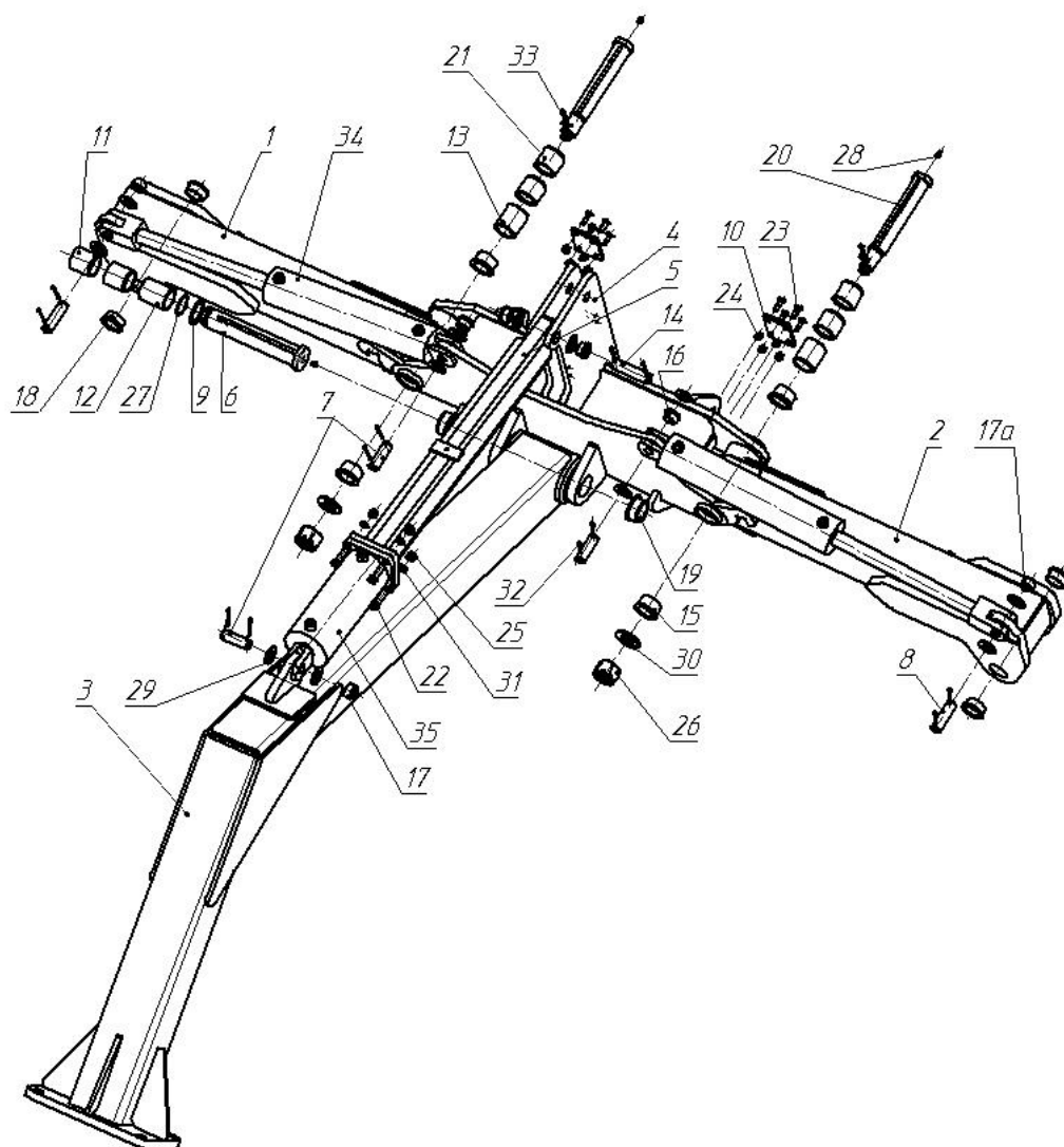
Рис.9 – КДК-6.02.000 Рама
