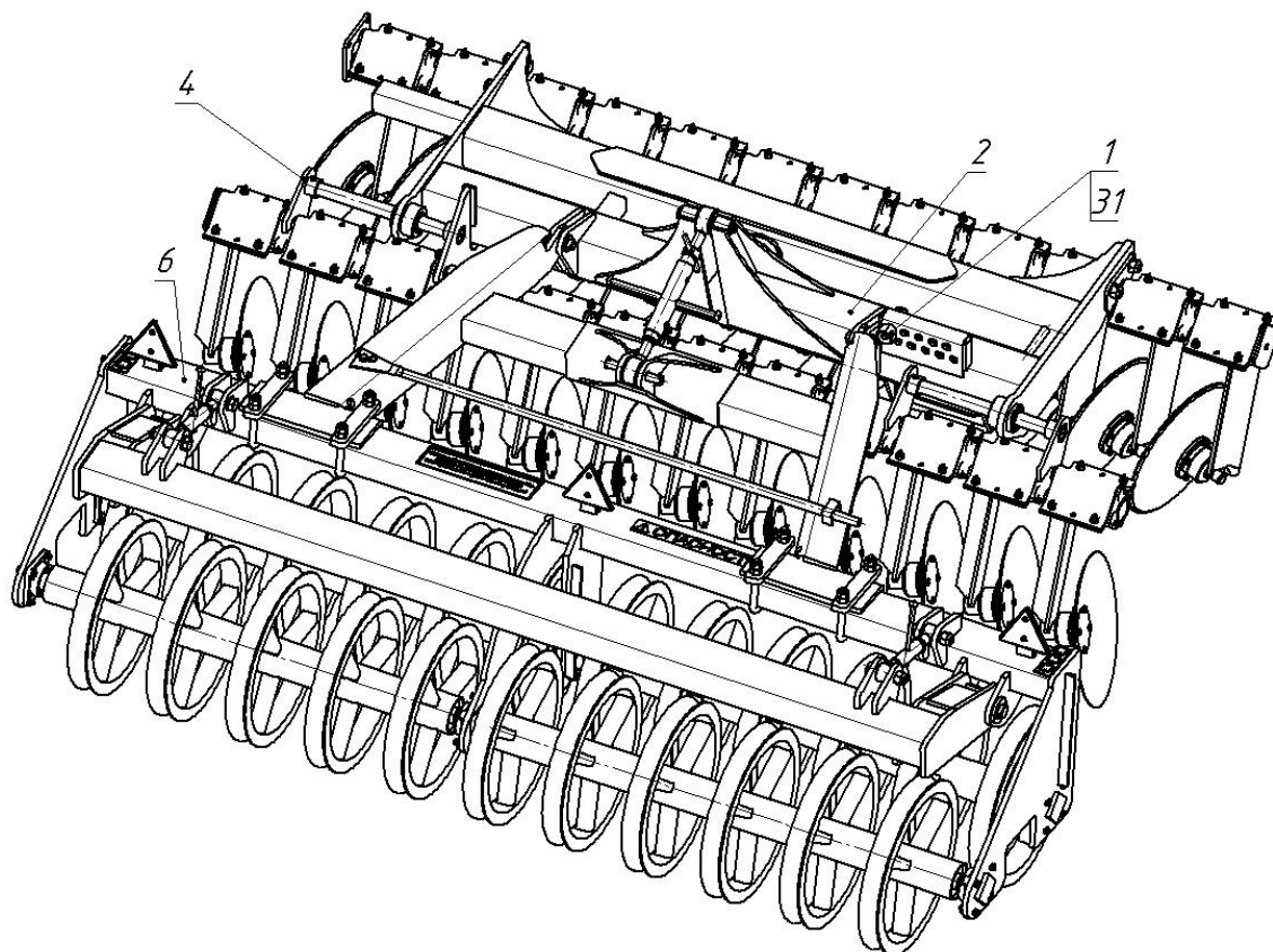
Рис.10.5 - КДК-6.03.000-05 СБ (с П-образным прикатчиком) (см. КДК-6.03.000 СБ)
