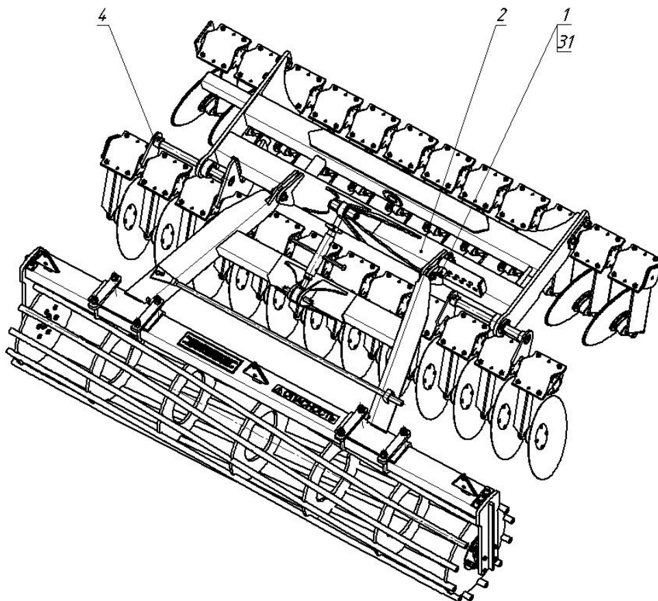
Рис.10.1 - КДК-6.03.000-01 СБ (с трубчатым прикатчиком) (см. КДК-6.03.000 СБ)
