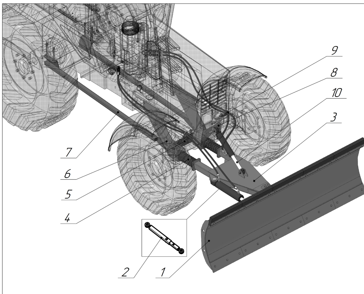
Рис. 1.1 Состав отвала
