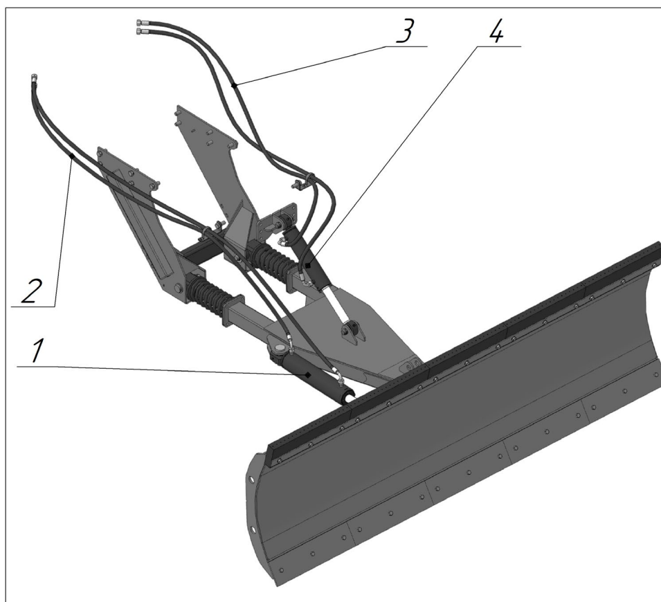
Рис. 1.2 Гидросистема отвала
