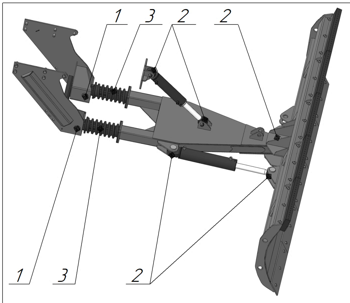
Рис. 3.1 Места нанесения смазочных материалов
