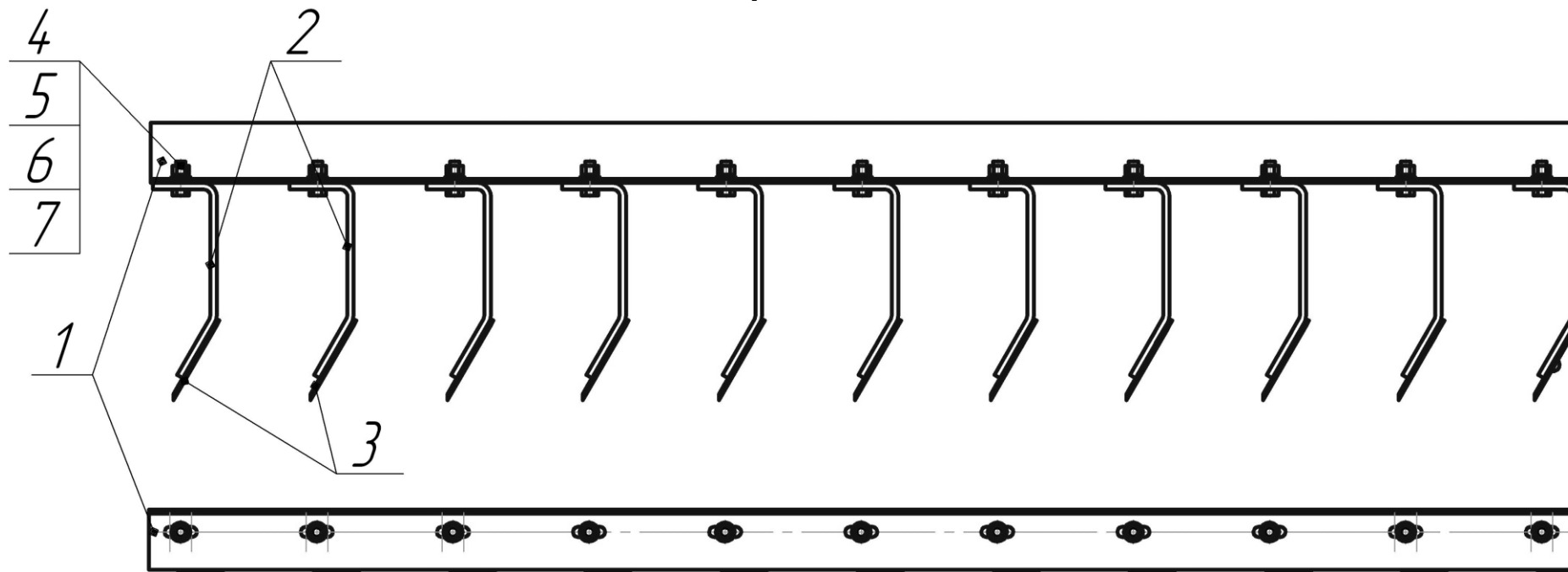
Схема расположения чистиков
