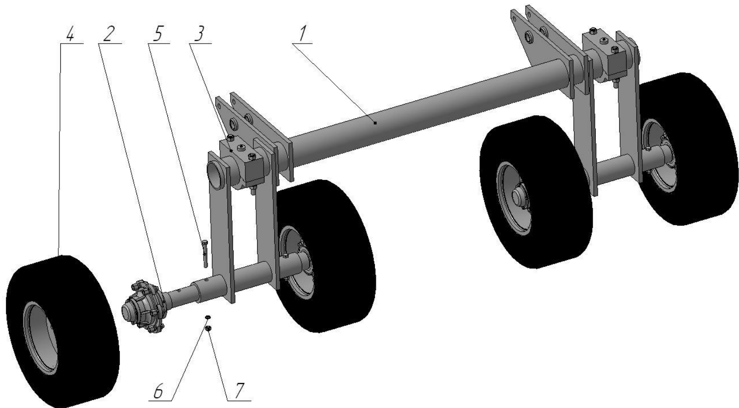
Колесная пара бороны БДЛП 8,0.
