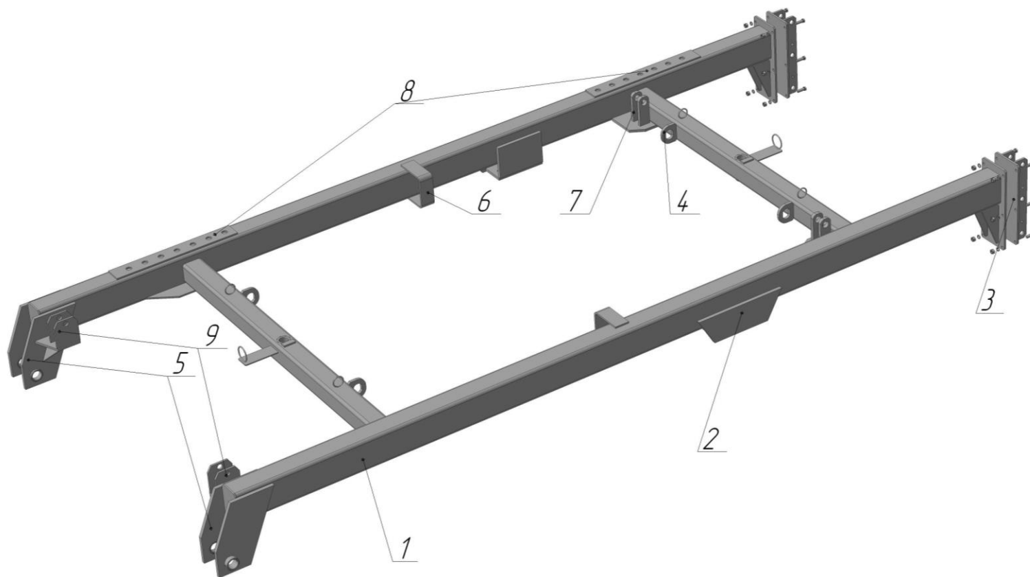
Рама дисковой бороны серии БДЛП 8,0 Катал. № БЛ801
