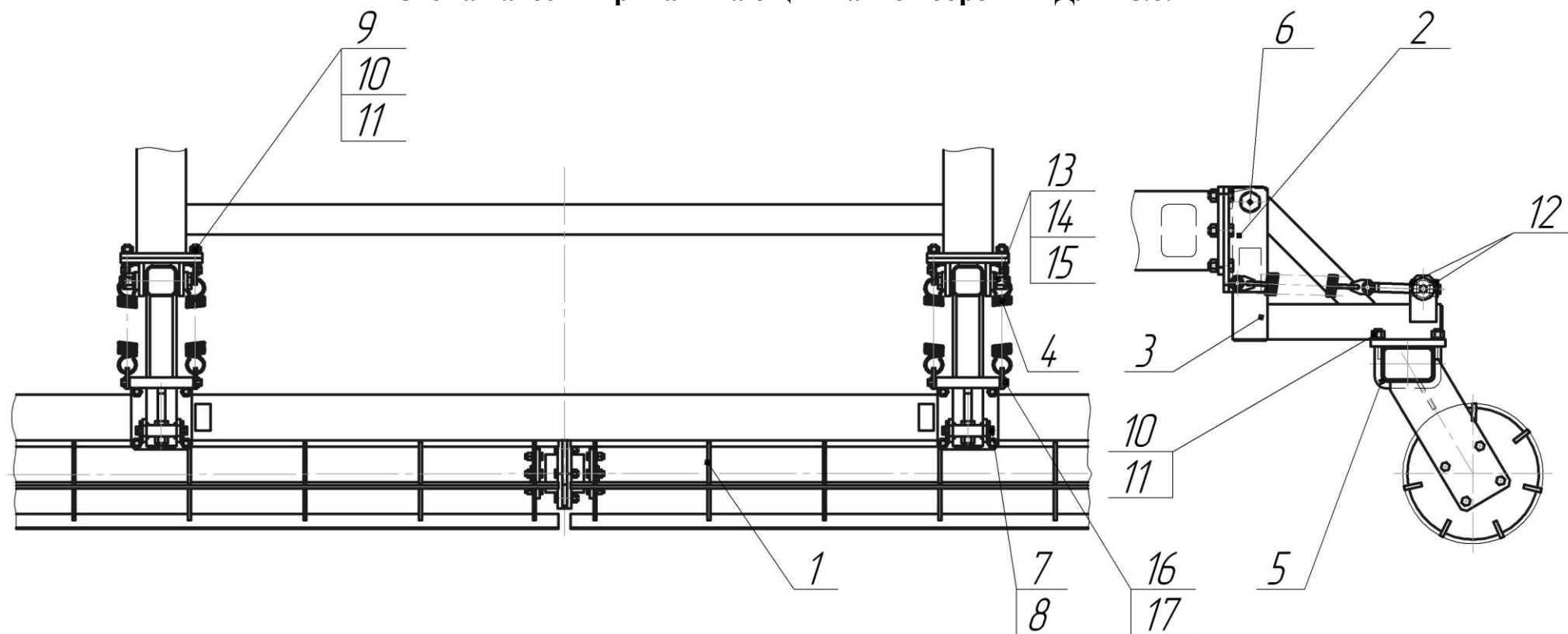
Схема навески прикатывающих катков бороны БДЛП-8.0.
