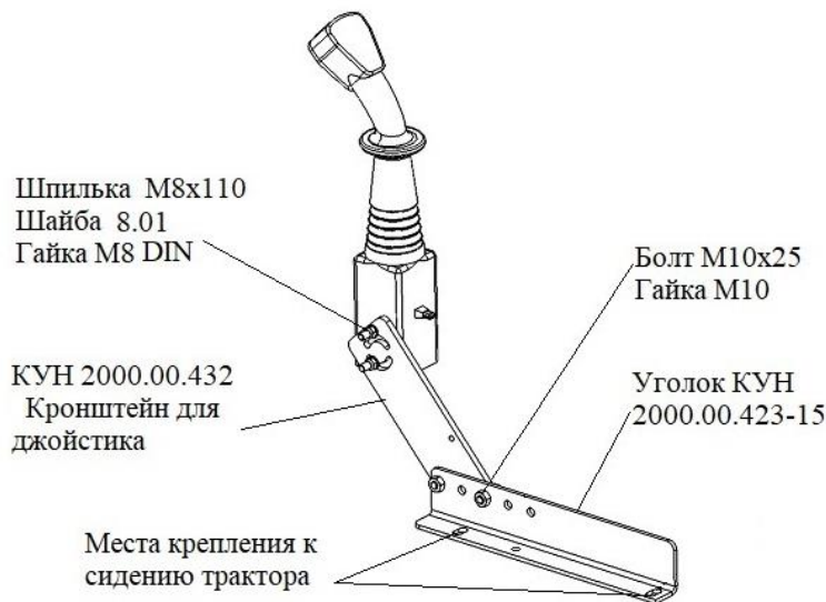
Рис.5 Установка уголка и джойстика
