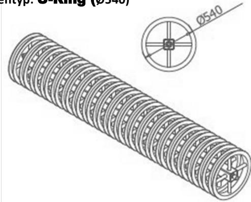
Walzentyp: U-Ring (Ø540)
