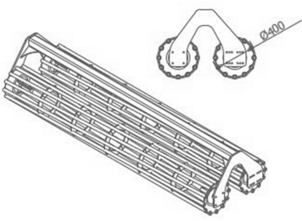
Walzentyp: DOPPELROHR (Ø400)
