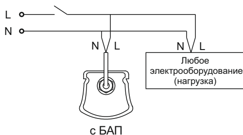
Рисунок 2 — Схема подключения светильника
