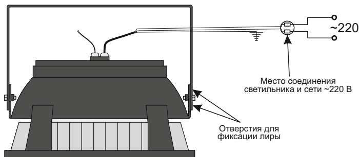
Рисунок 2 — Схема подключения изделия
