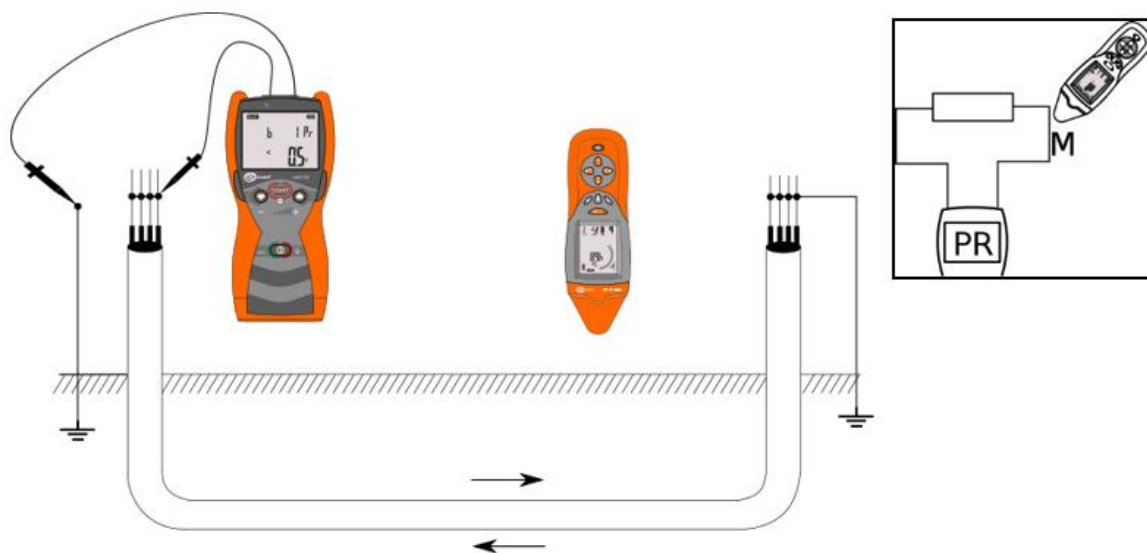
Поиск кабельной линии с замкнутыми жилами в режиме «мощность»
