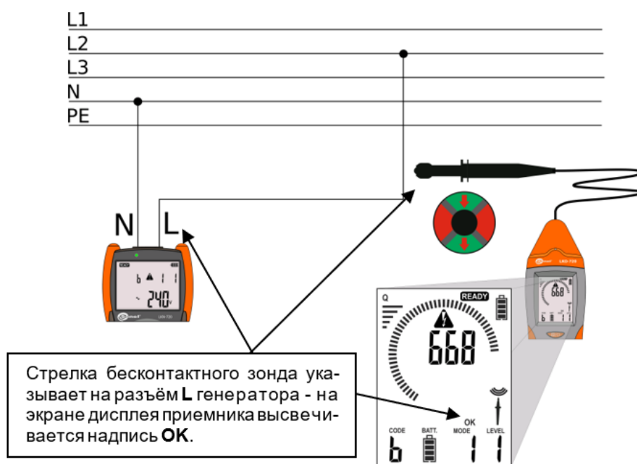
Идентификация разъёма L генератора
