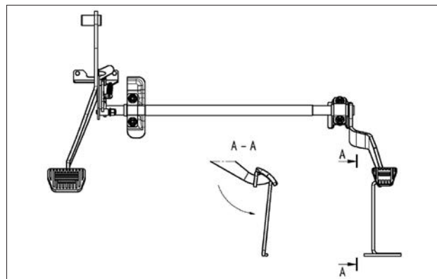
Схема для автоматической коробки передач
