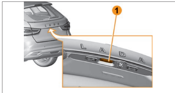
Рис. 1.6.3. Открытие крышки/двери багажного отделения (в варианном исполнении)
