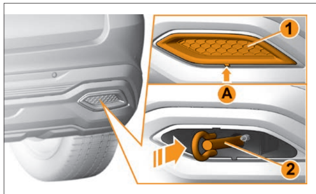
Рис. 6.13.2. Установка буксирной проушины в заднем бампере
