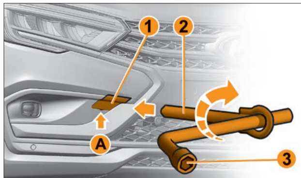
Рис. 6.13.1. Установка буксирной проушины в переднем бампере
