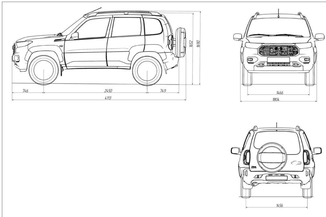
Рис. 85. Габаритные (справочные) размеры автомобиля (в варианном исполнении)
