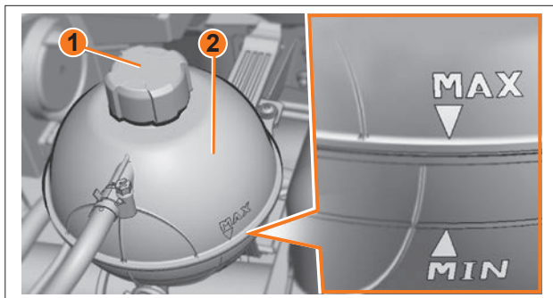
Рис. 70. Проверка уровня охлаждающей жидкости в расширительном бачке
