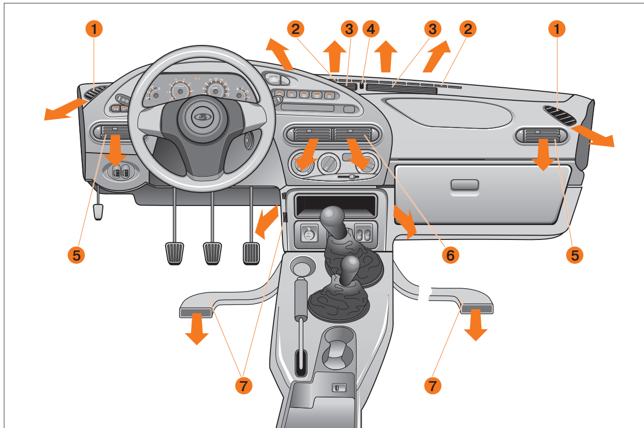
Рис. 47. Распределение потоков воздуха системы вентиляции и отопления салона
