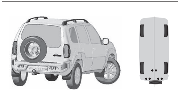
Рис. 34. ТСУ и точки его крепления (в вариантном исполнении)
