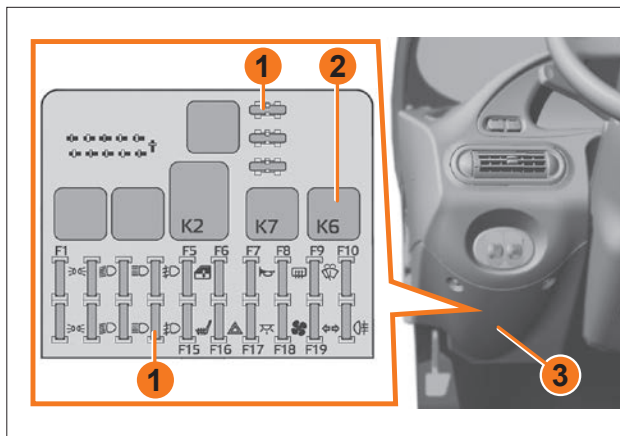
Рис. 79а. Монтажный блок – схема установки (для автомобиля со светодиодными блок-фарами)
