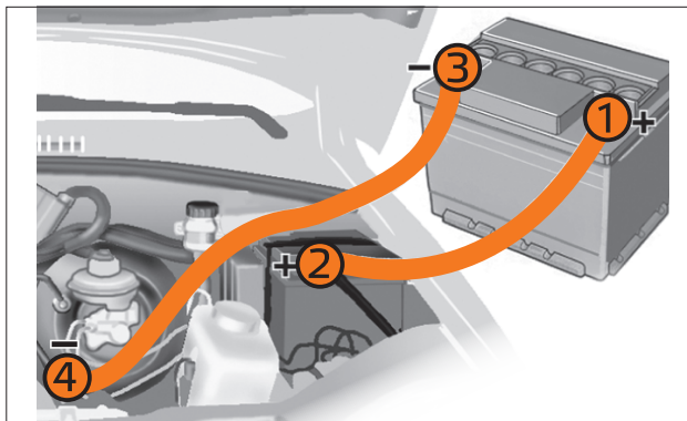
Рис. 62. Схема подключения пусковых проводов к вспомогательной батарее
