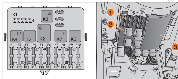
Рис. 79. Монтажный блок – схема установки (для автомобиля с галогеновыми блок-фарами)
