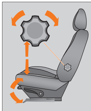
Рис. 14. Рукоятки регулировки сиденья (в варианном исполнении)
