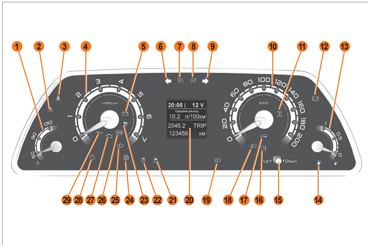
Рис. 40а. Комбинация приборов
