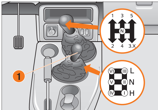
Рис. 46. Положение рычагов трансмиссии
