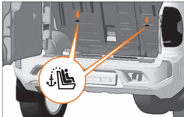
Рис. 26. Расположение верхнего страховочного ремня ISOFIX
