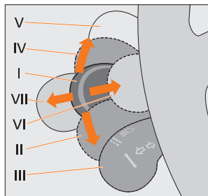
Рис. 42. Подрулевые переключатели
