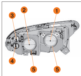
Рис. 80. Блок-фара
