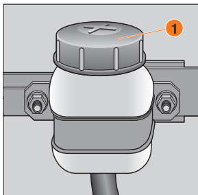
Рис. 72. Бачок гидропривода выключения сцепления
