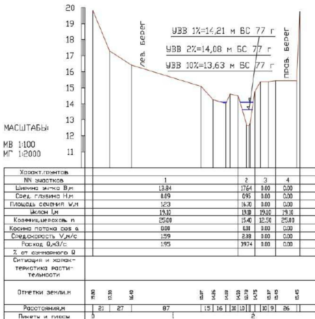
Рисунок 7 –График морфостроения через руч. Сухой
