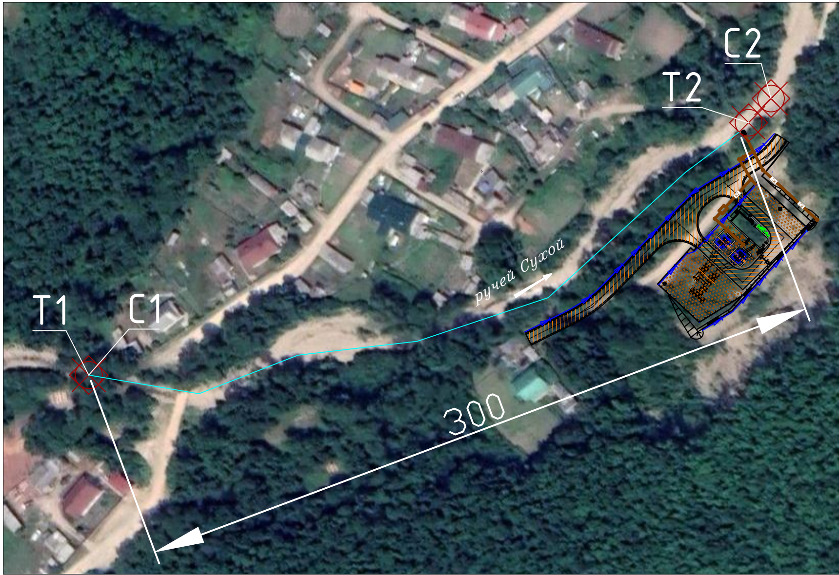
Рисунок 2 – Схема планировочной организации земельного участка ПС 35 кВ Терней
