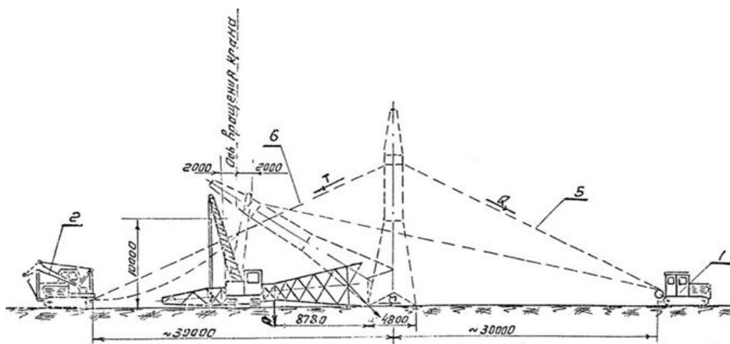
Р и с у н о к 5 - Установка опоры ВЛ
