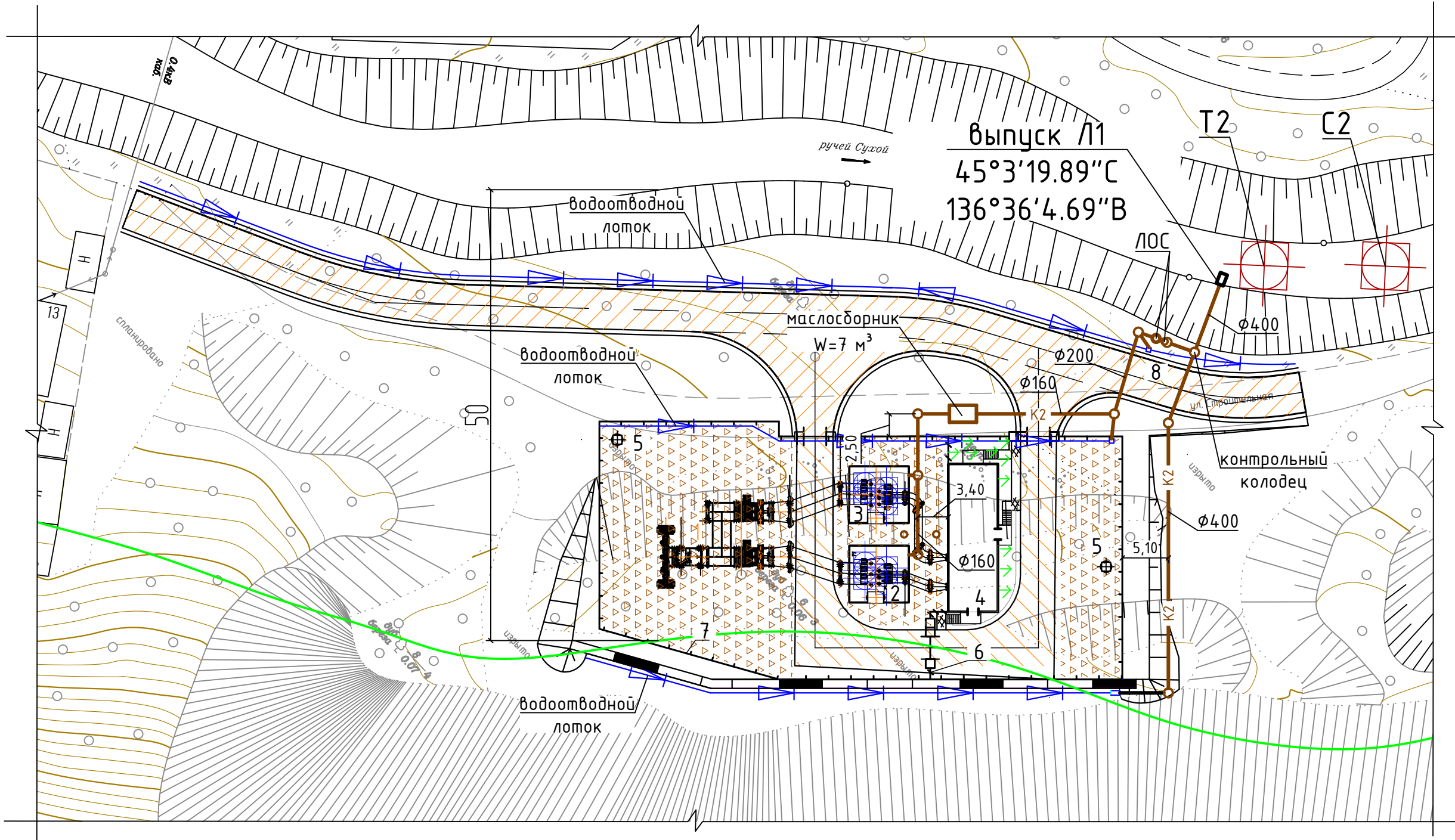
Рисунок 2 – Схема планировочной организации земельного участка ПС 35 кВ Терней
