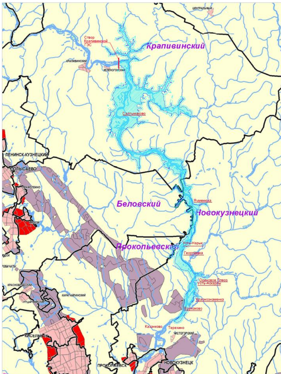
Рисунок 2 – Карта-схема Крапивинского водохранилища при НПУ 177,50 м с обозначением поселений, затрагиваемых при реализации варианта ТП 1976 г.
