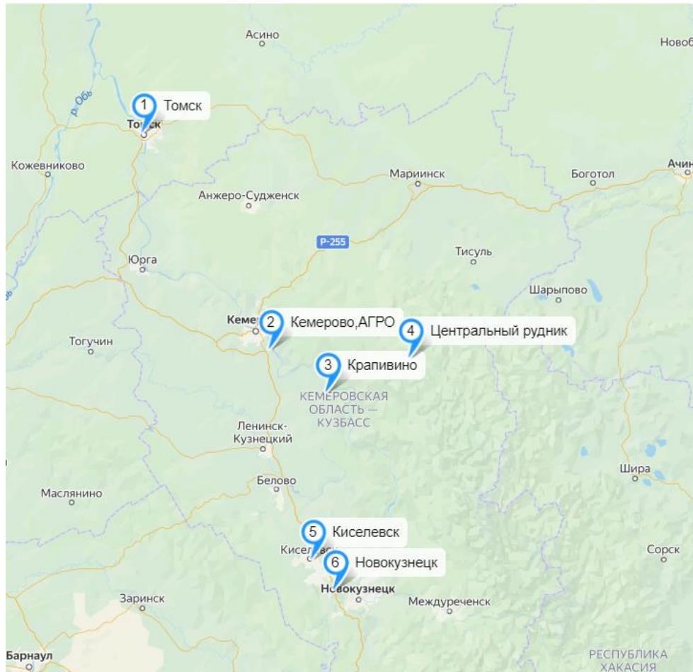
Рисунок 3 - Схема расположения метеостанций, используемых для анализа климата района Крапивинского водохранилища
