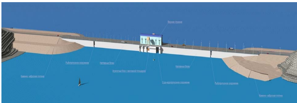
Компоновка сооружений проектируемой Северной ПЭС
