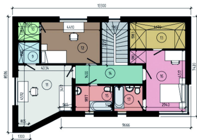
Экспликация помещений
