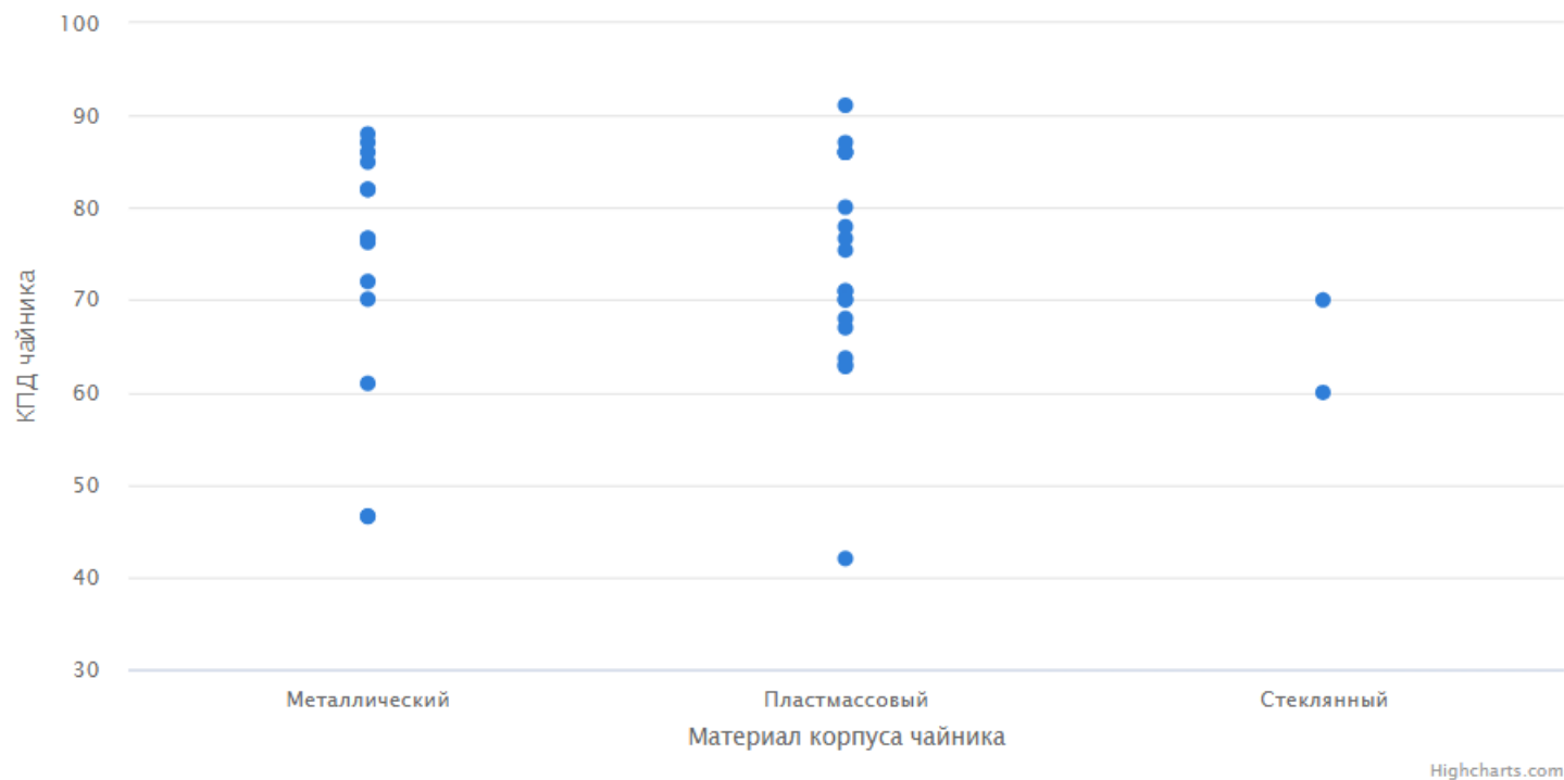
Зависимость КПД чайника от материала его корпуса
